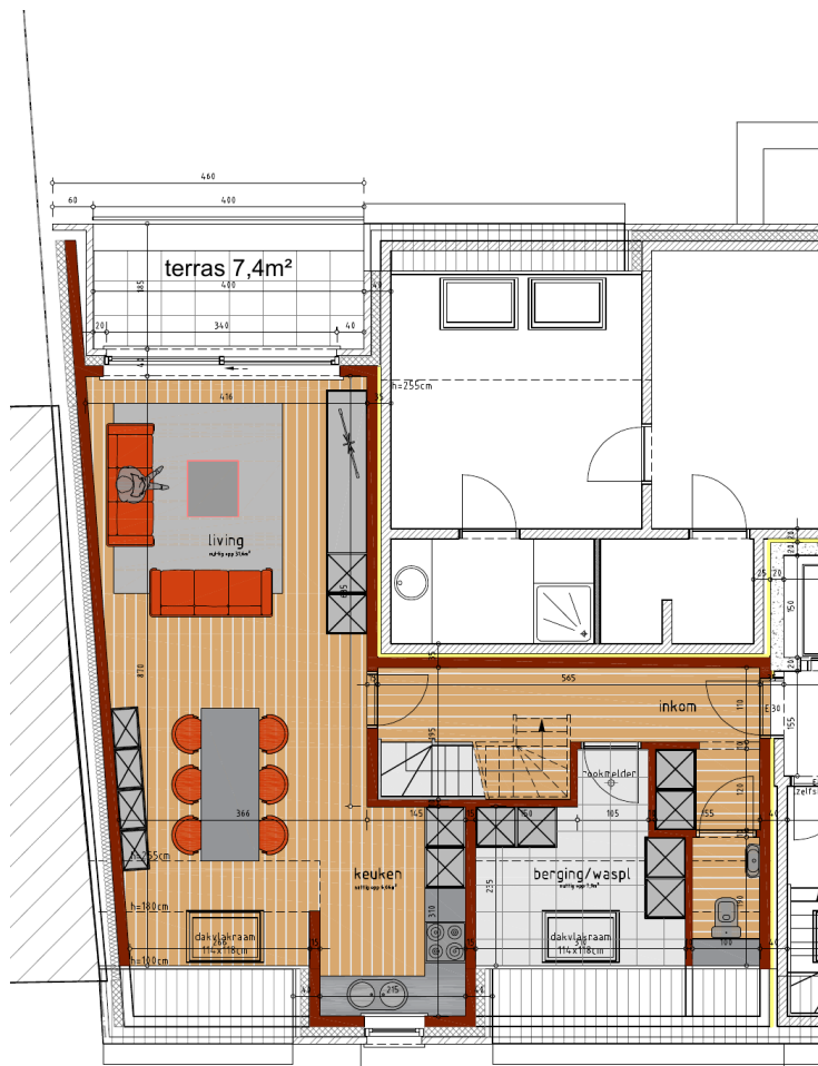
2e verdieping
