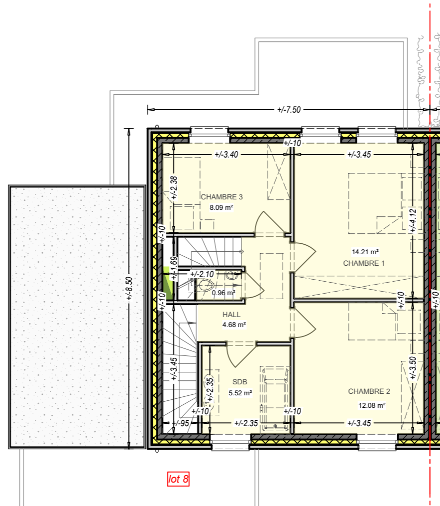
PLAN ETAGE
