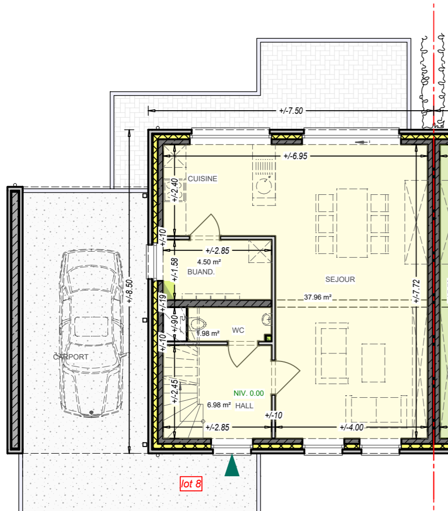
PLAN REZ-DE-CHAUSSEE
