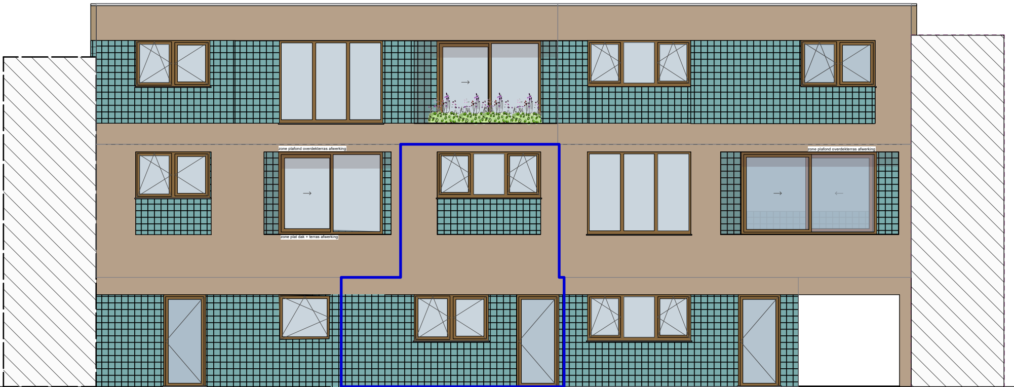
Voorgevel
