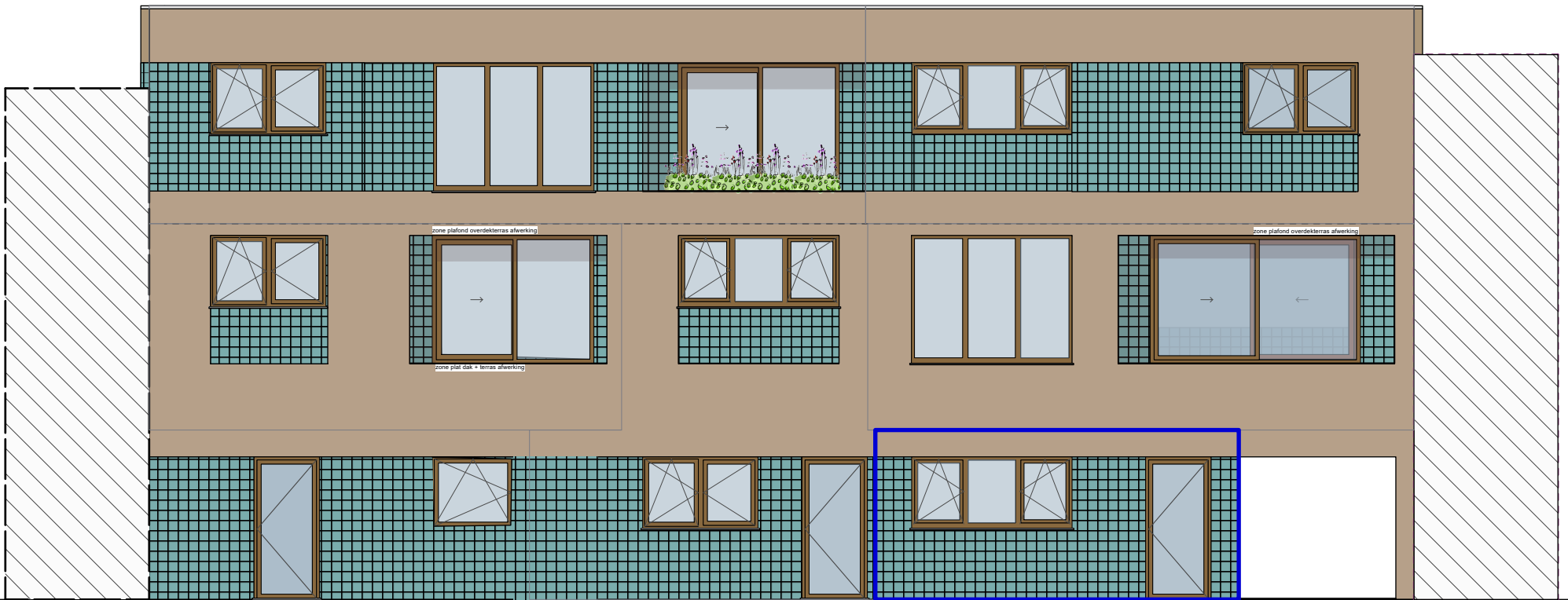
Voorgevel
