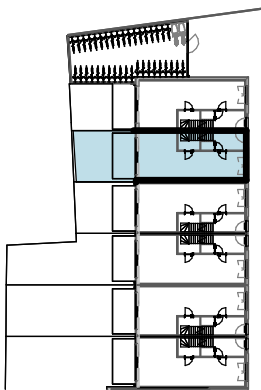
Gelijkvloers Inplanting
