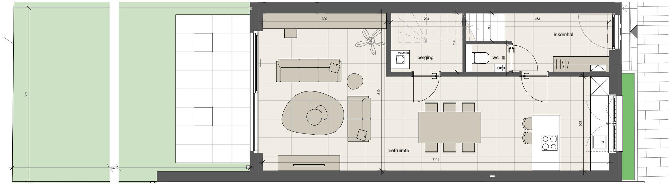
Gelijkvloers 1:75
