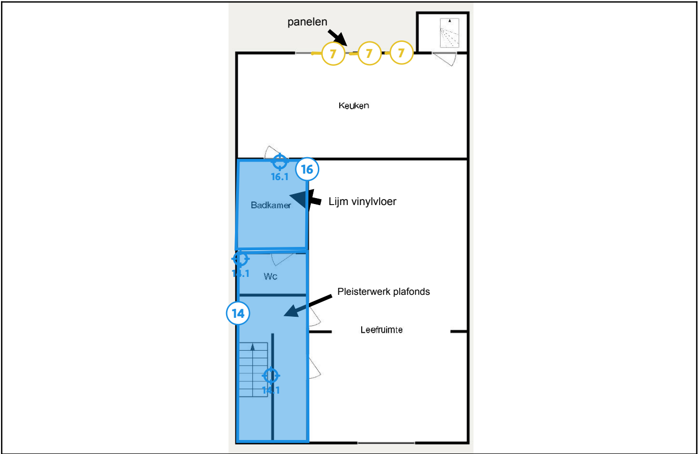
Legende van plan 1.4: Grondplan +1: pleister plafonds, panelen, lijm
