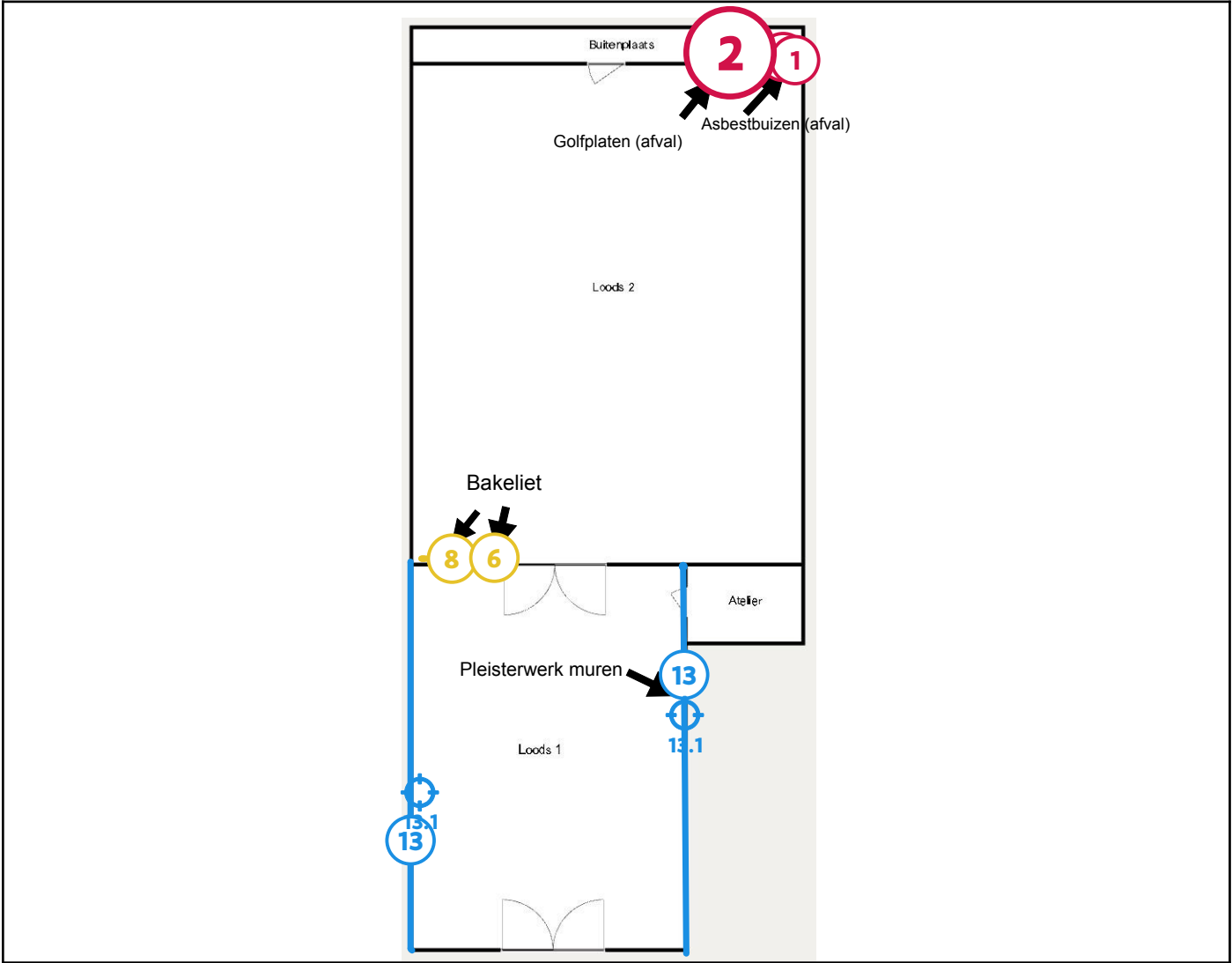
Legende van plan 1.2: Grondplan 0: golfplaten,buis, bakeliet, pl.muren
