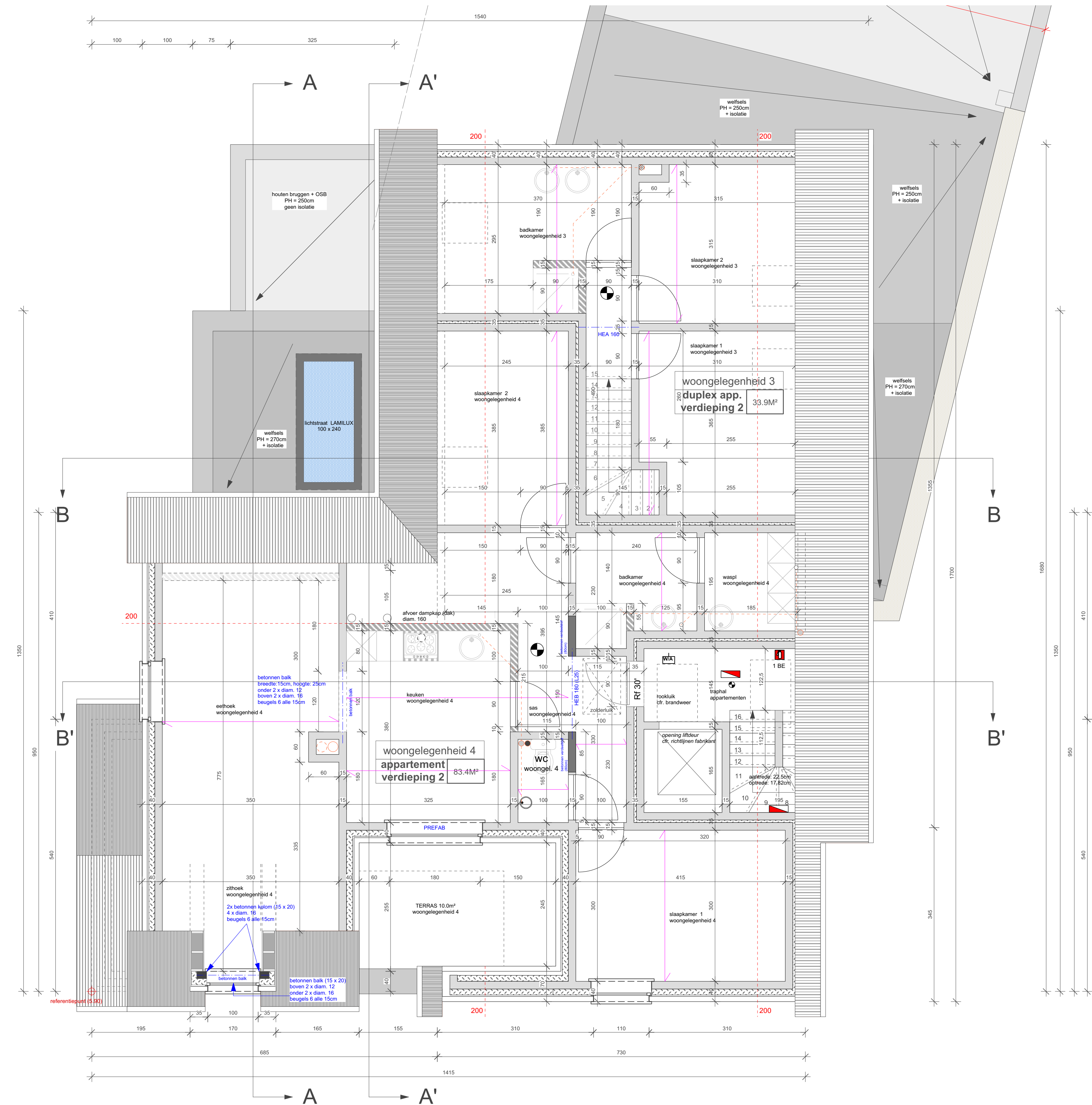
VERDIEPING 2 1/50
