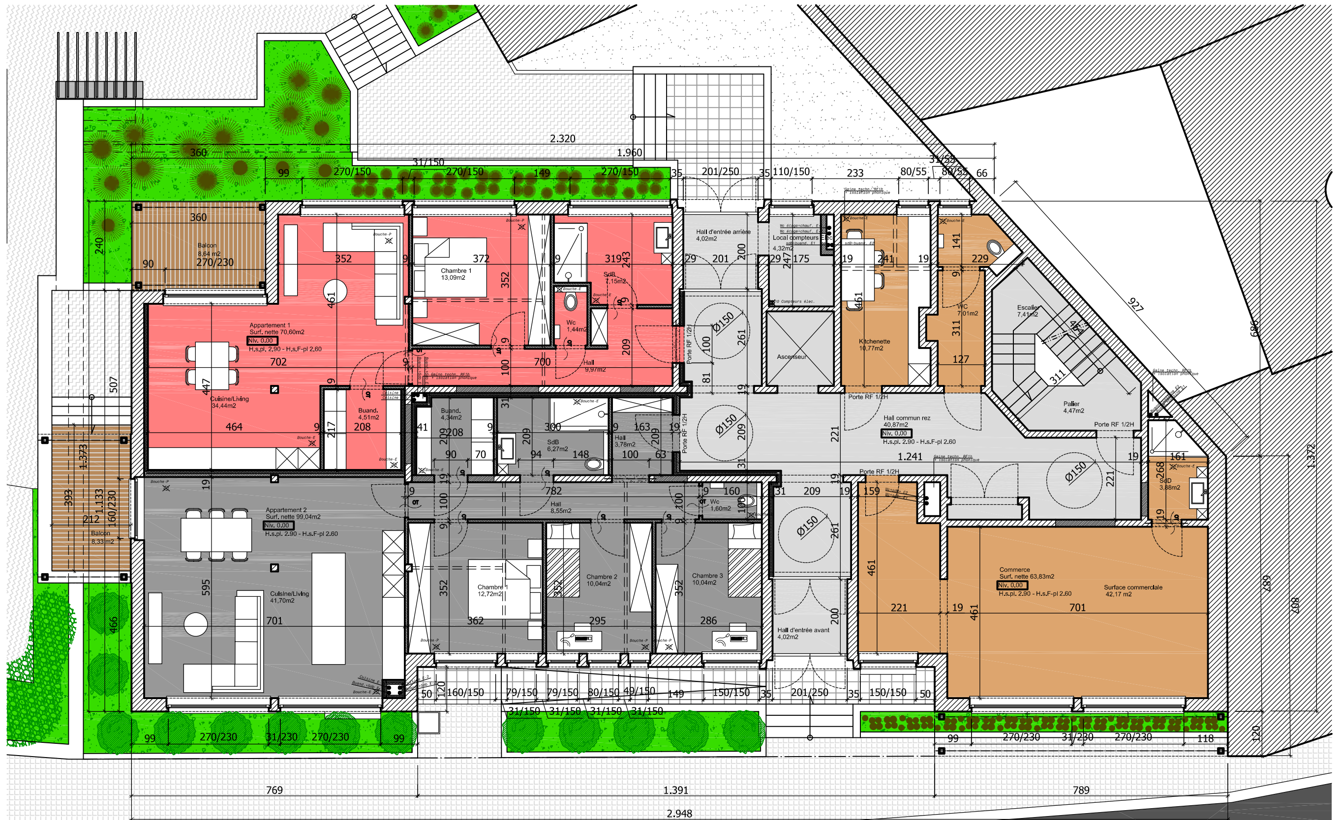
Vue en plan Rez-de-chaussée – Projeté Ech.: 1/100
