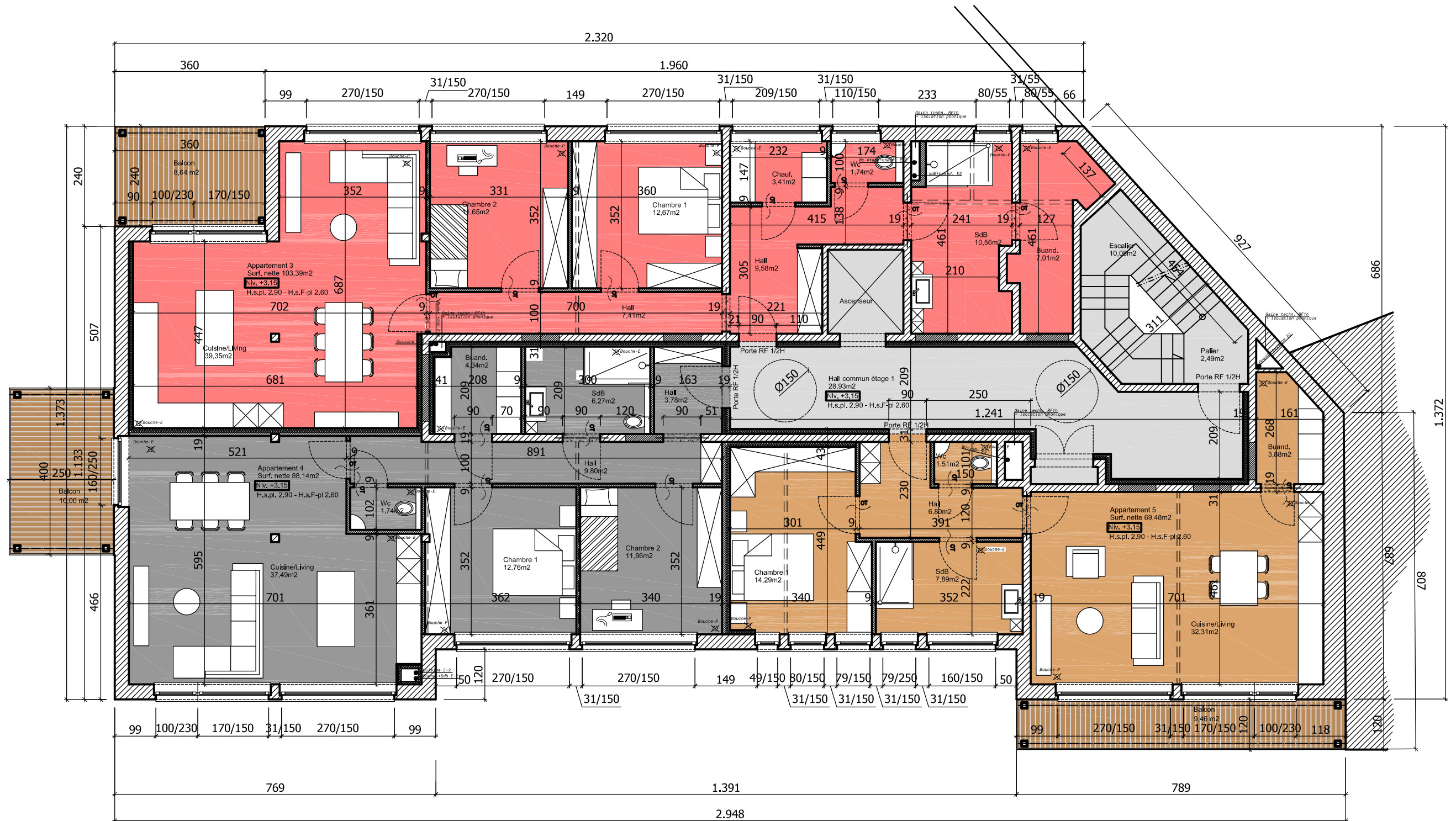
Vue en plan Etage 1 – Projeté Ech.:1/100
