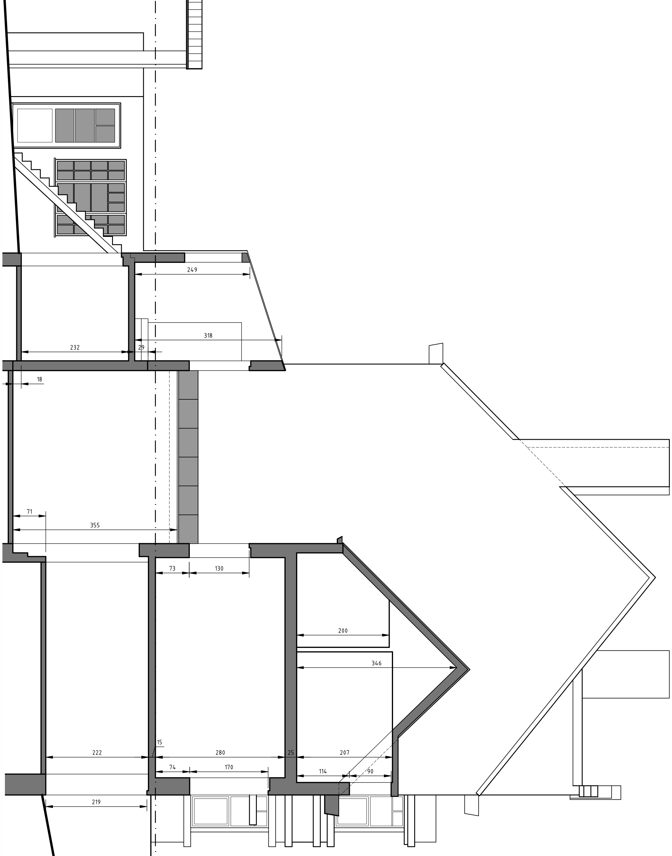
COUPE BB
