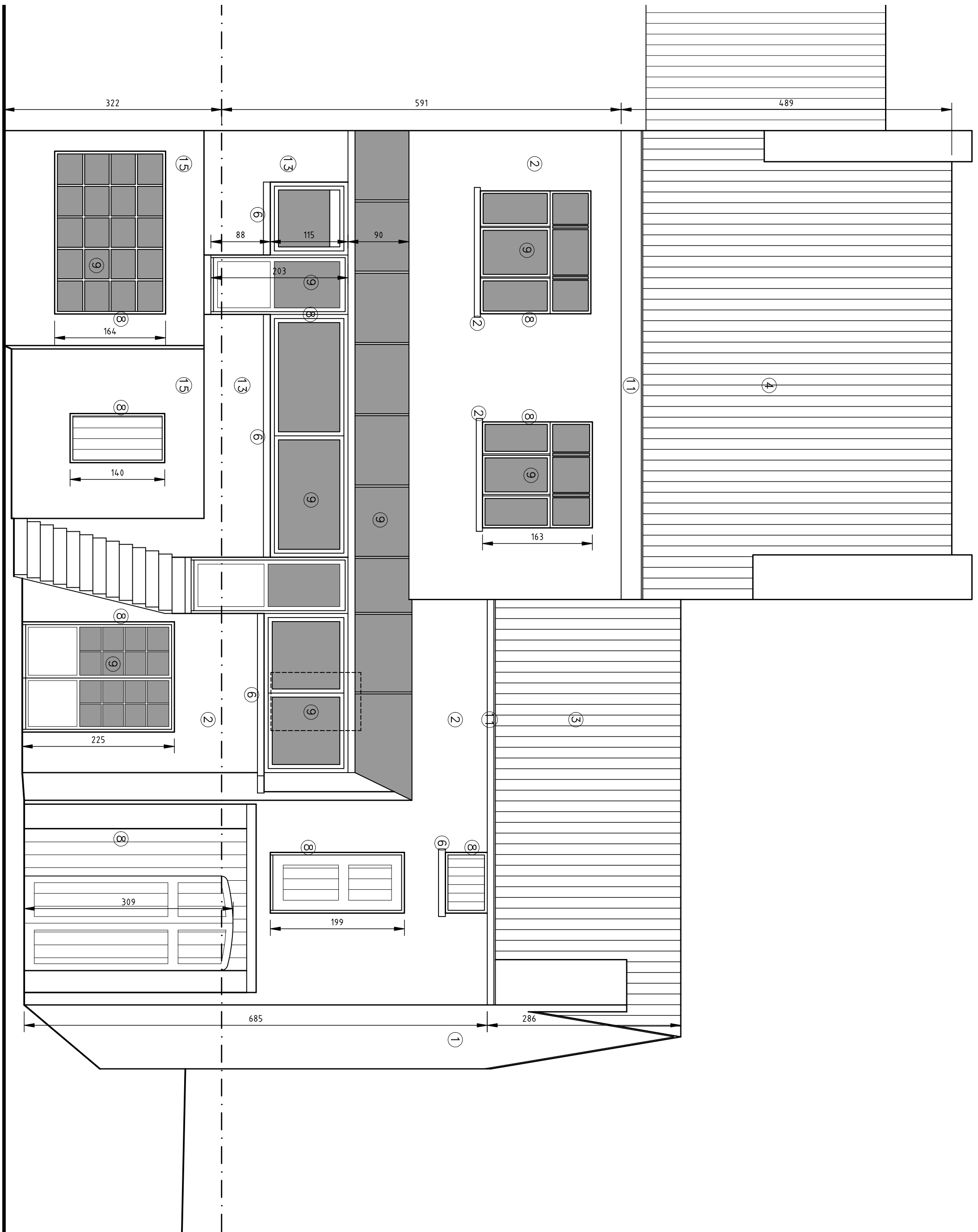
FACADE ARRIÈRE
