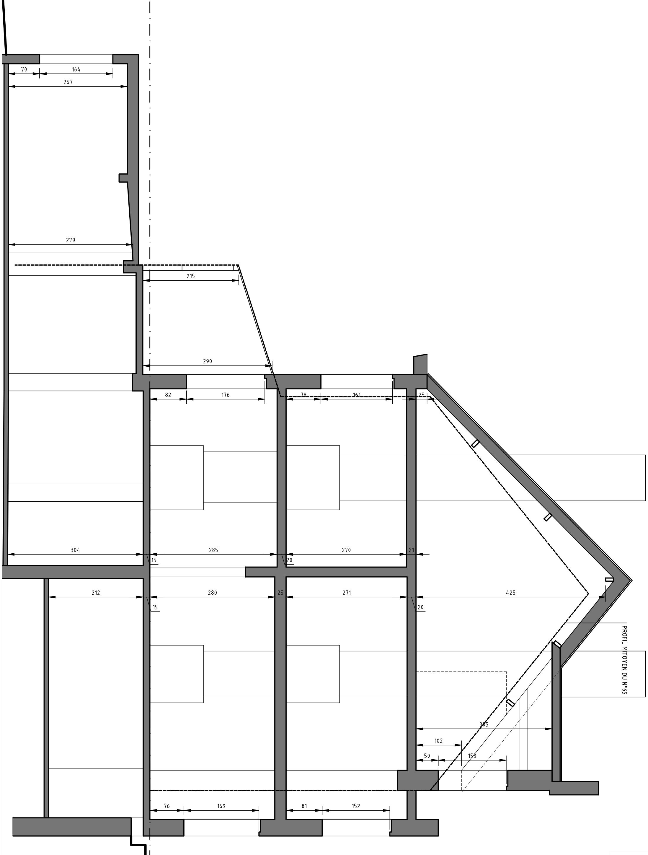
COUPE AA
