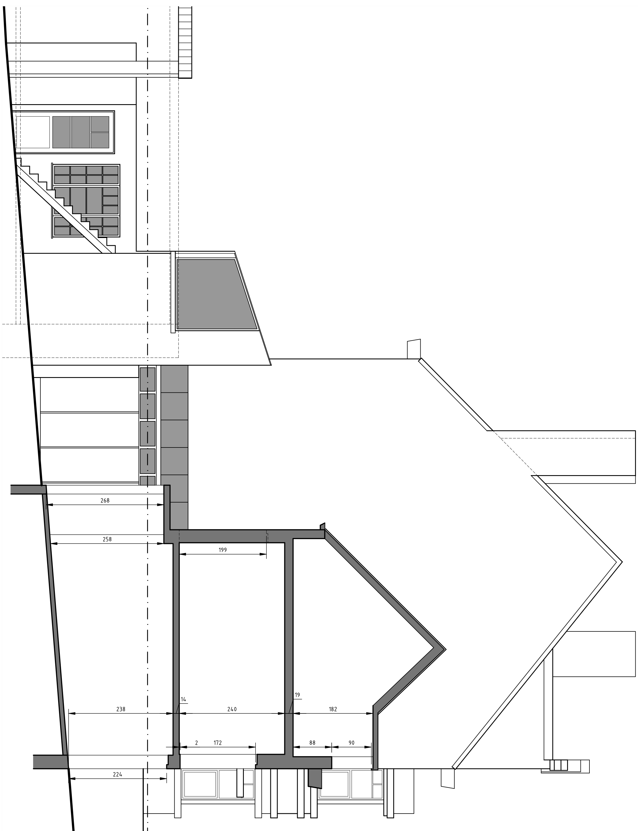
COUPE CC
