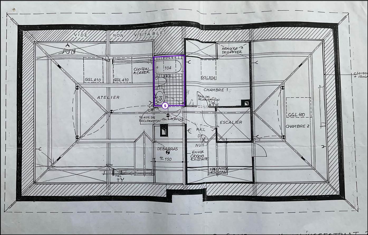
Legende van plan 1.3: 1ste verdiep
