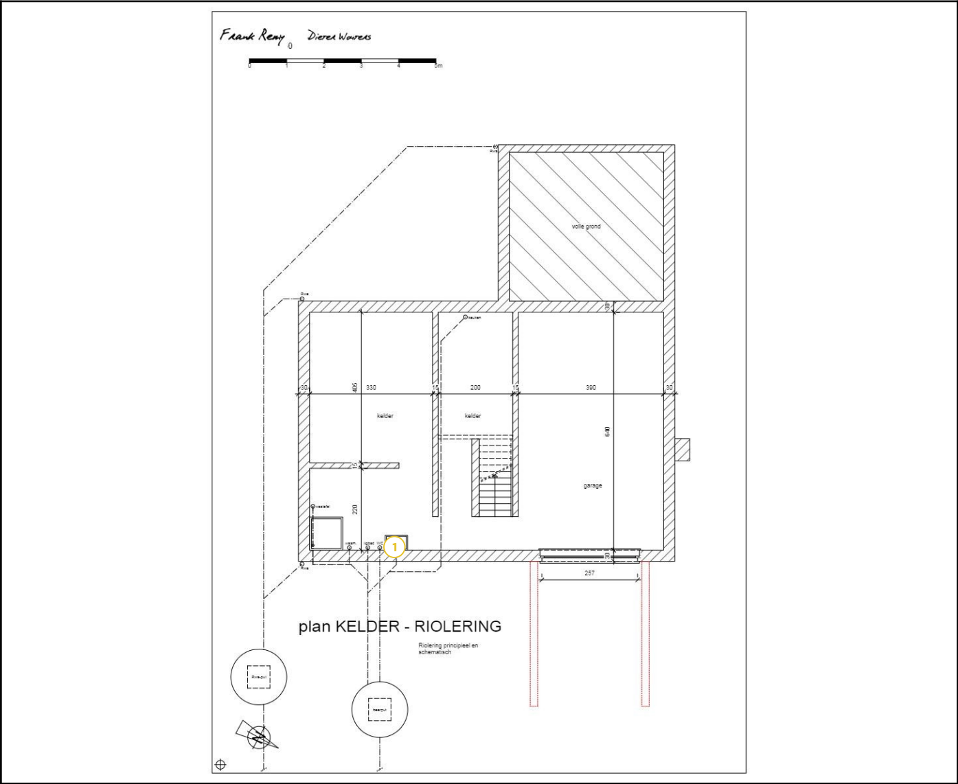
Legende van plan 1.3: Kelder en garage; meterkast
