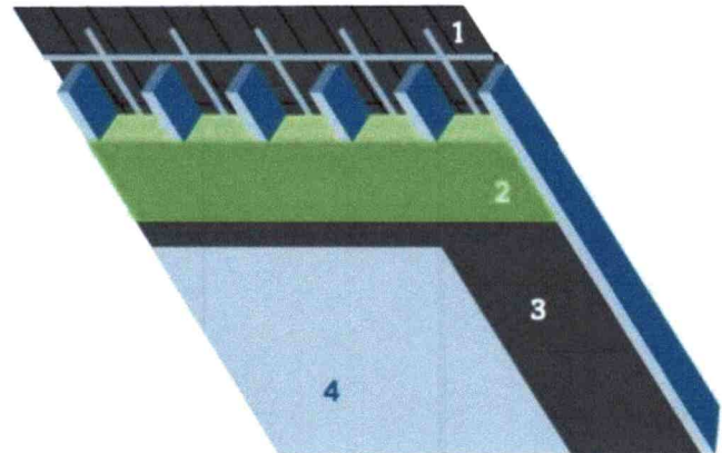
1. Onderdak | 2. Isolatie | 3. Dampscherm | 4. binnenafwerking
