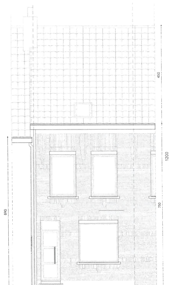
VOORGEVEL (bestaand en ongewijzigd)
