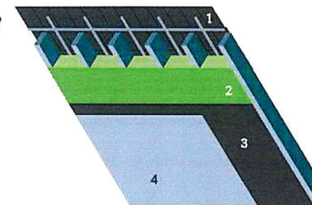
1. Onderdak | 2. Isolatie | 3. Dampscherm | 4. binnenafwerking
