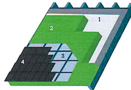
1. Dampscherm | 2. Isolatie | 3. Onderdak | 4. Dakbedekking
