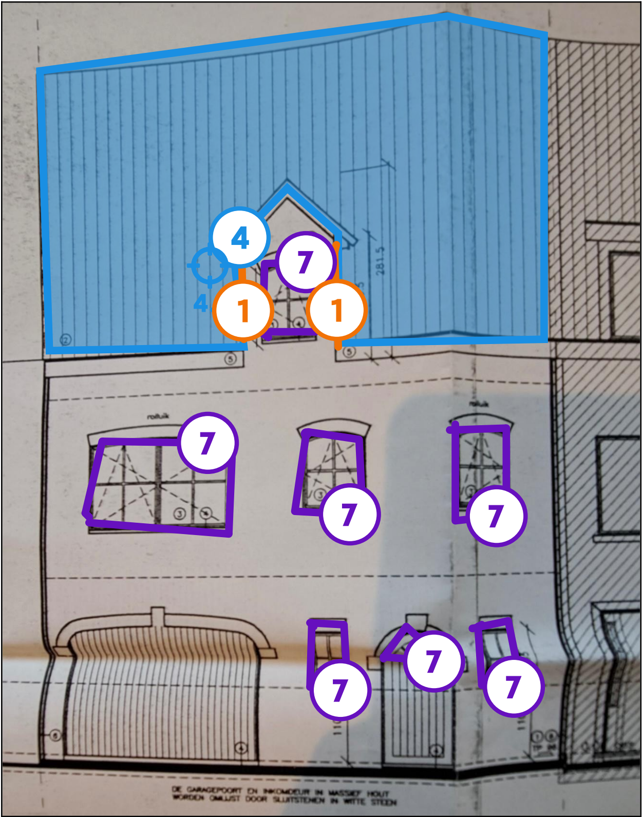
Legende van plan 1.4: Voorgevel
