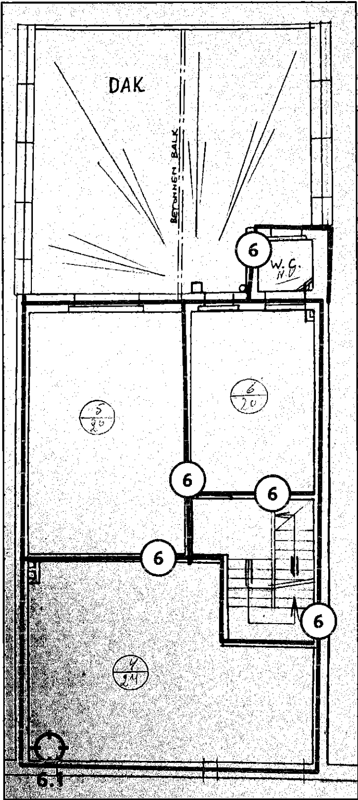
Legende van plan 1.3: Plan 1e verdiep muren
