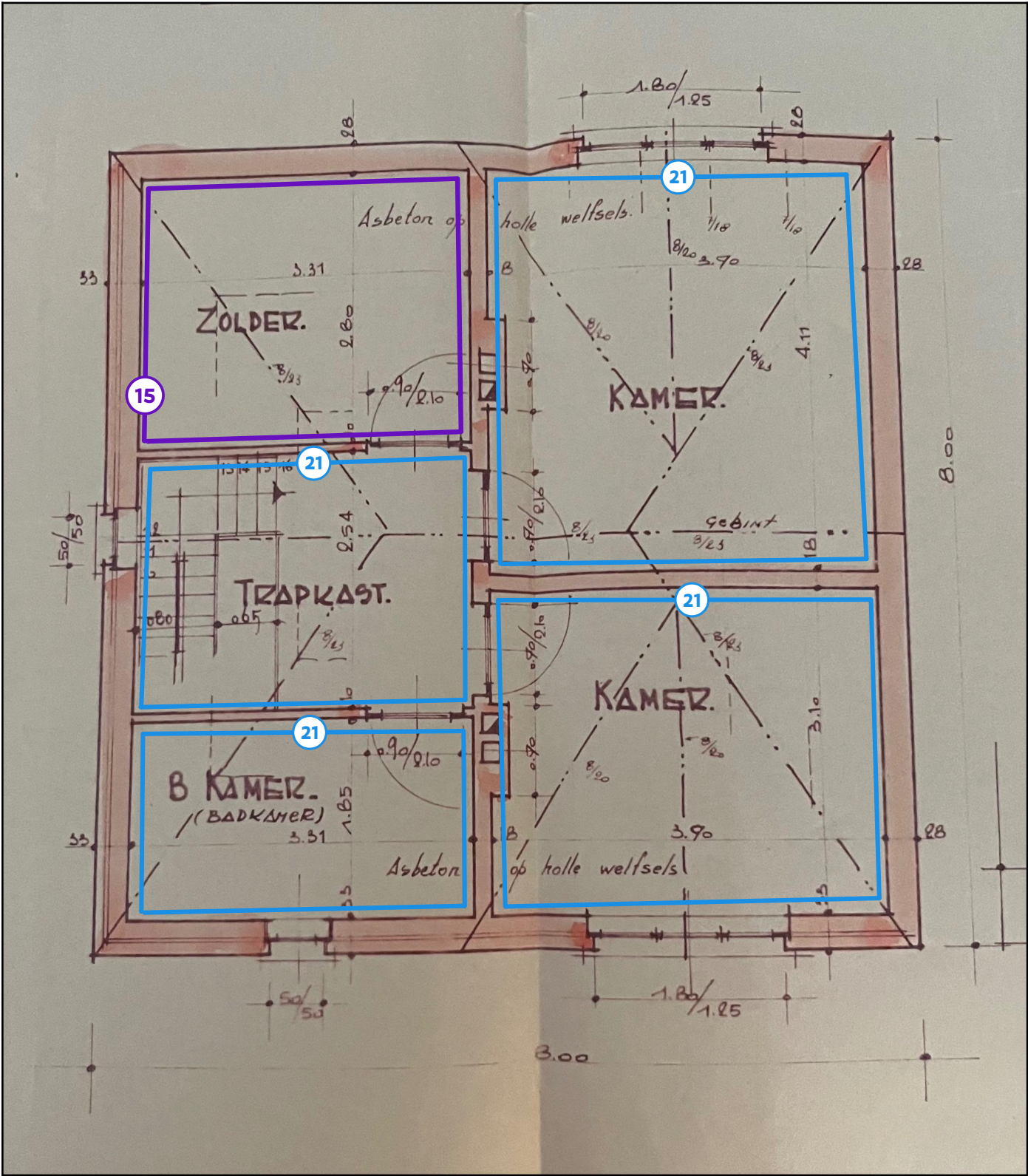
Legende van plan 1.6: Eerste verdieping
