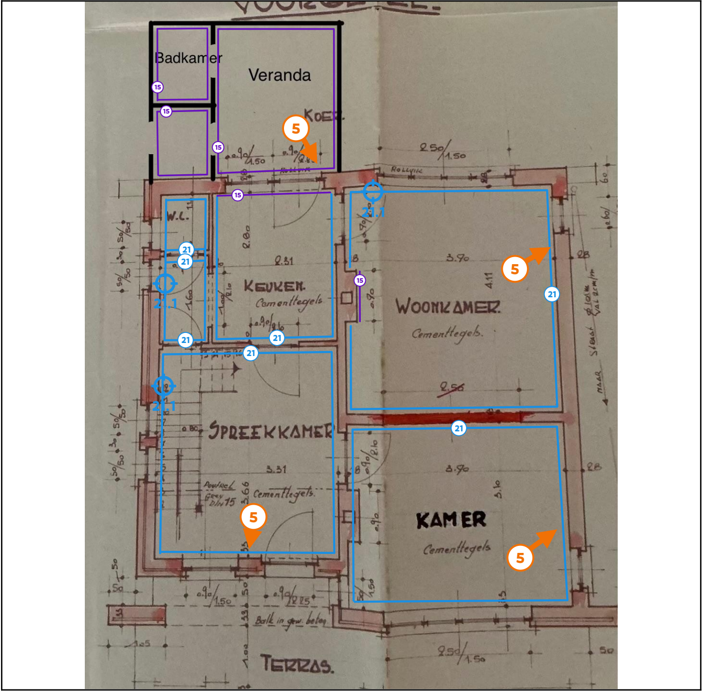
Legende van plan 1.1: Gelijkvloers woongedeelte
