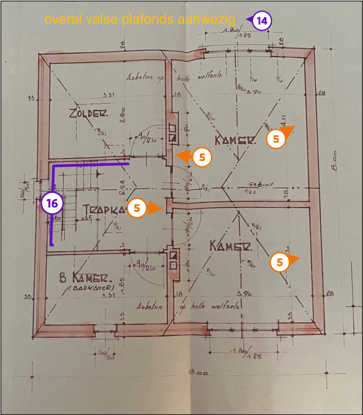
Legende van plan 1.7: Eerste verdieping
