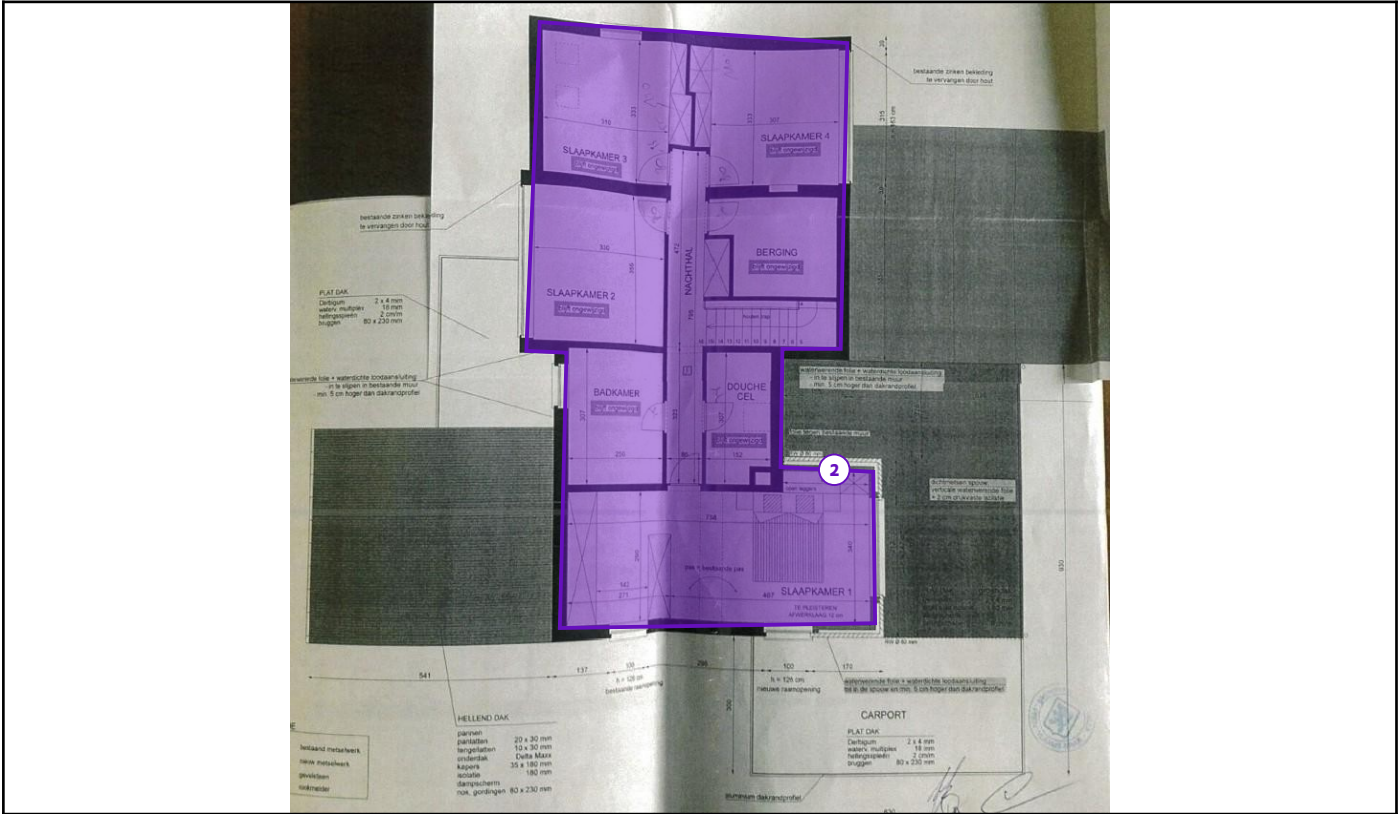
Legende van plan 1.5: Plan - 1ste verdieping
