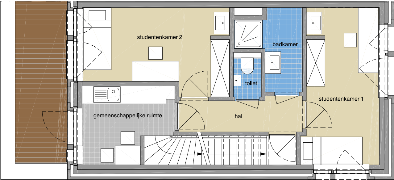
Verdieping +2
