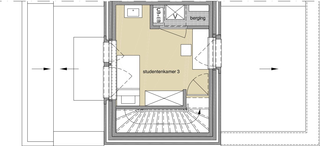
Verdieping +3
