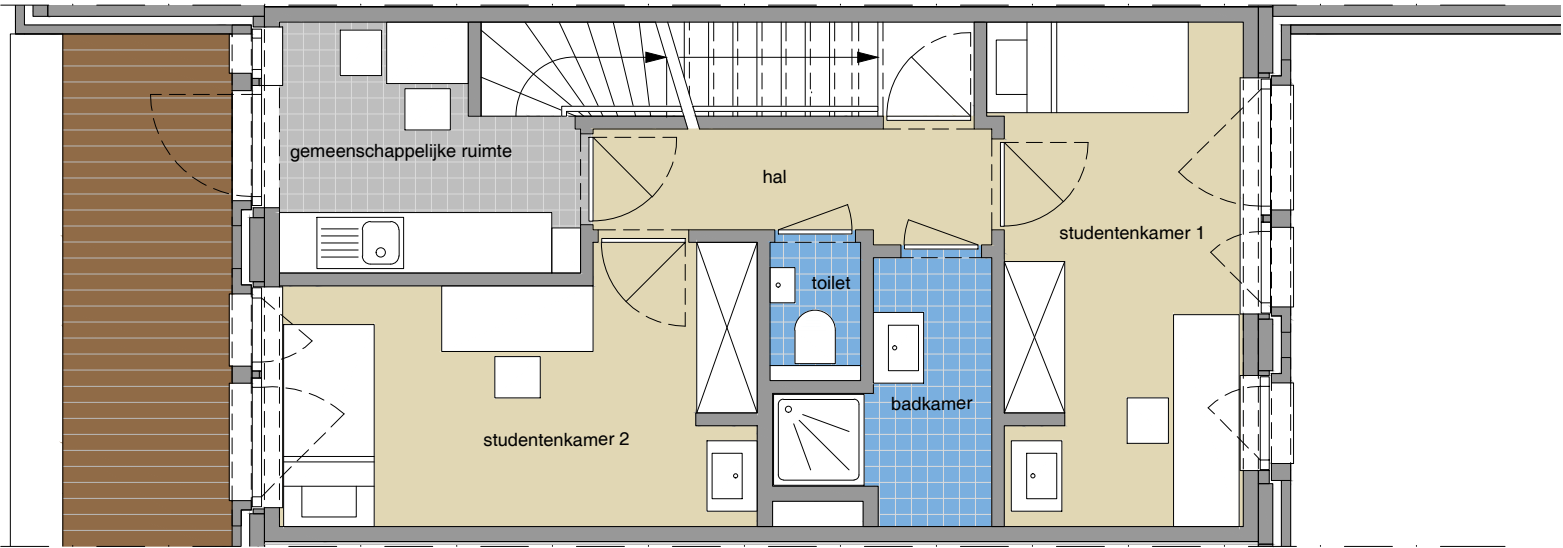
Verdieping +2
