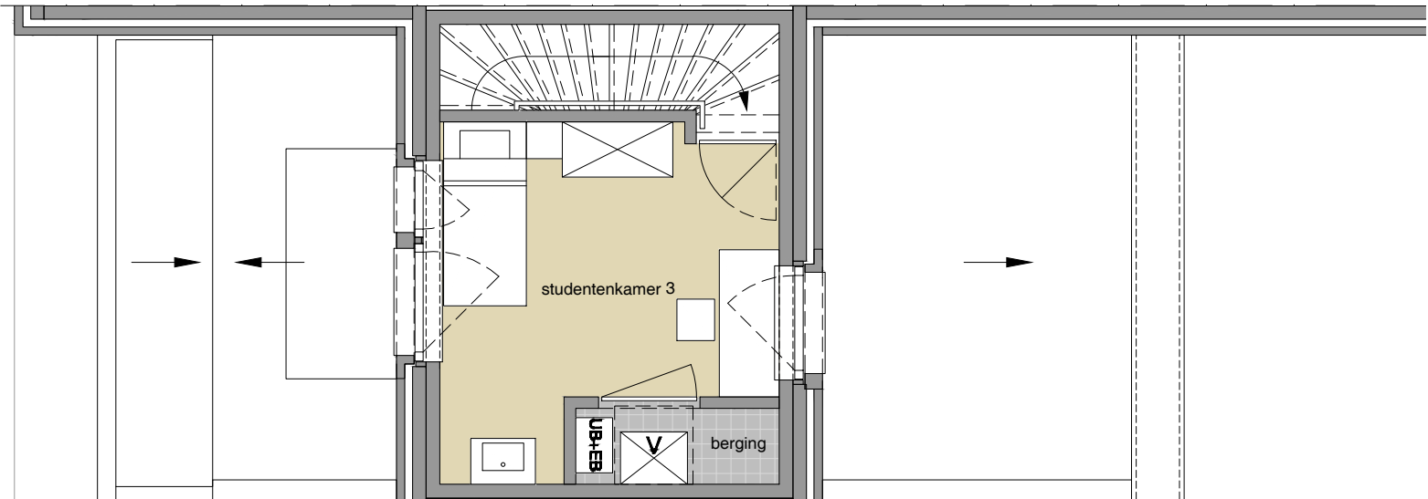
Verdieping +3
