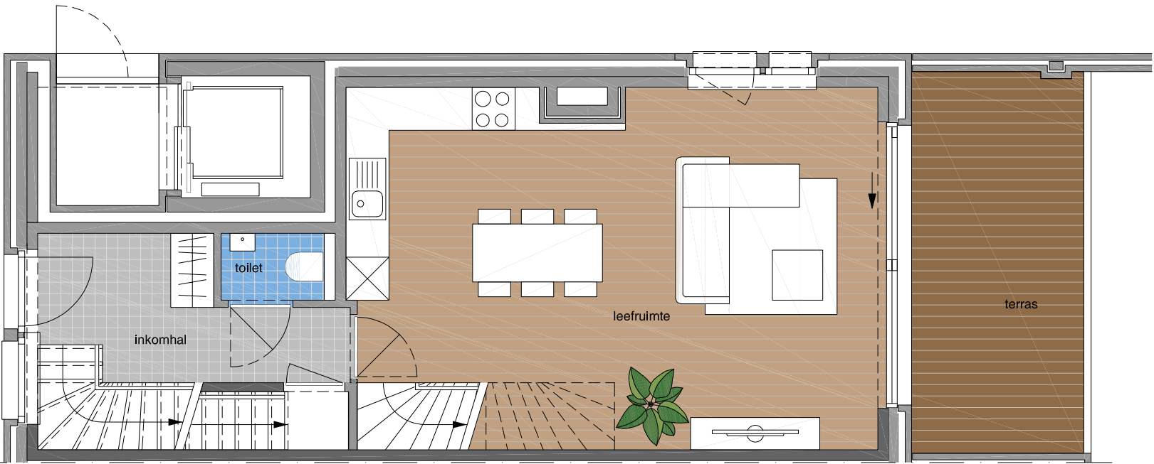
Gelijkvloerse verdieping
