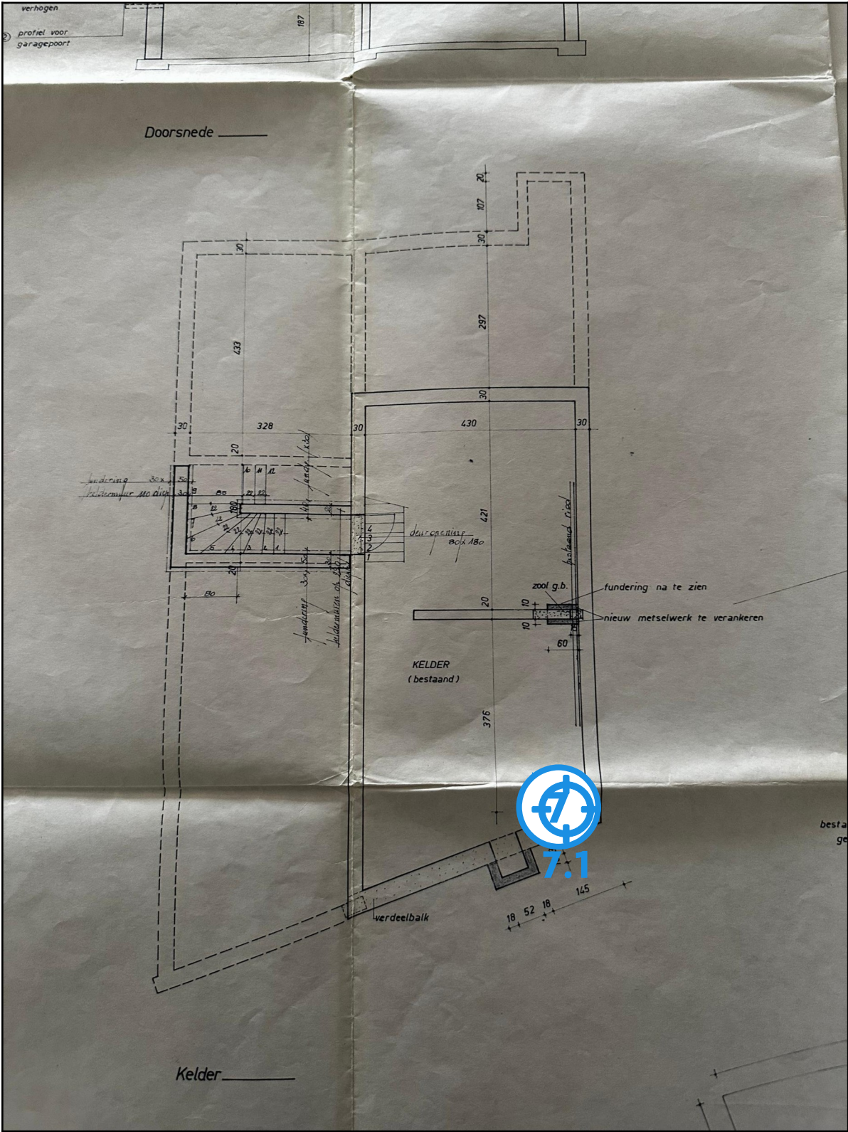
Legende van plan 1.1: Grondplan kelder
