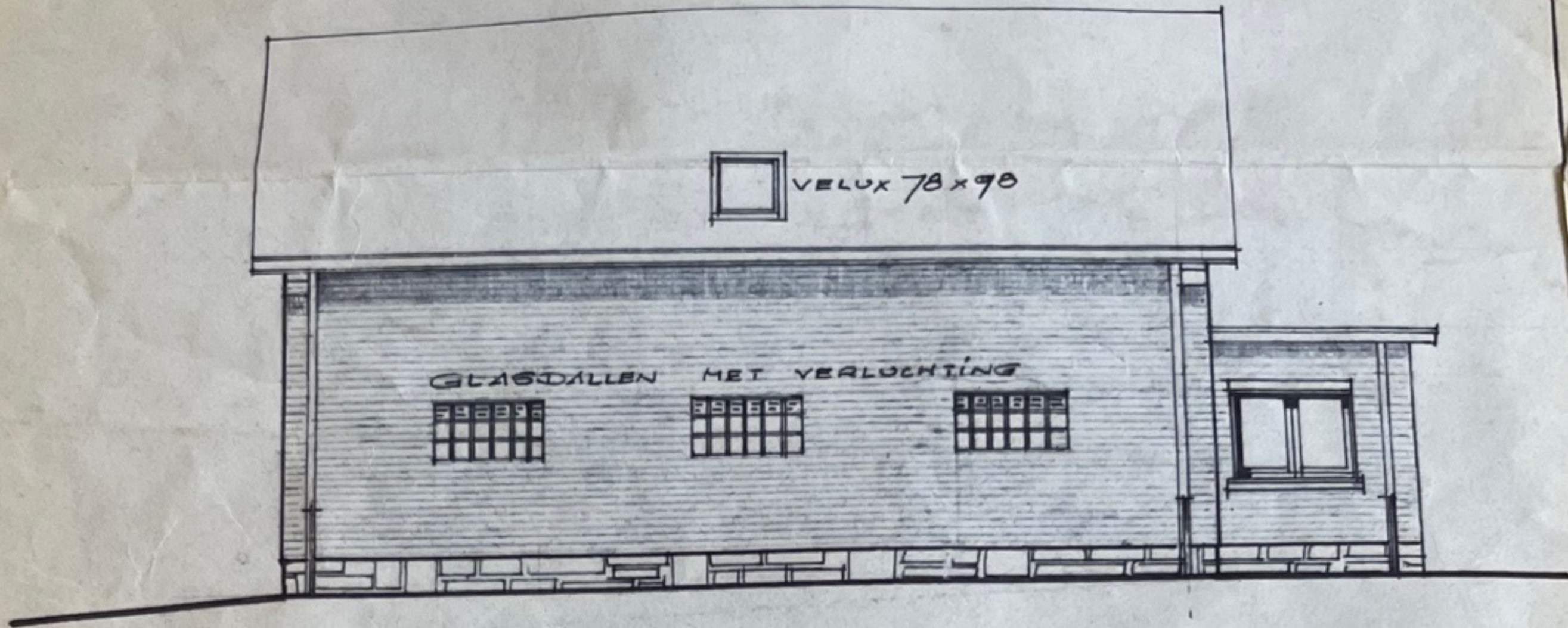
ZIJGEVEL RECHTS. 1/100
