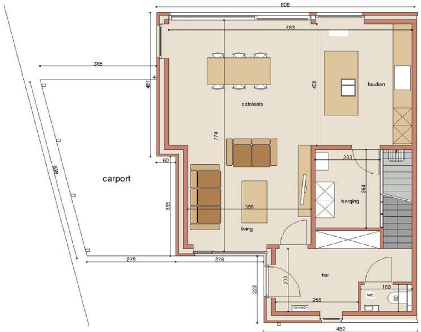
lot 3 gelijkvloers
