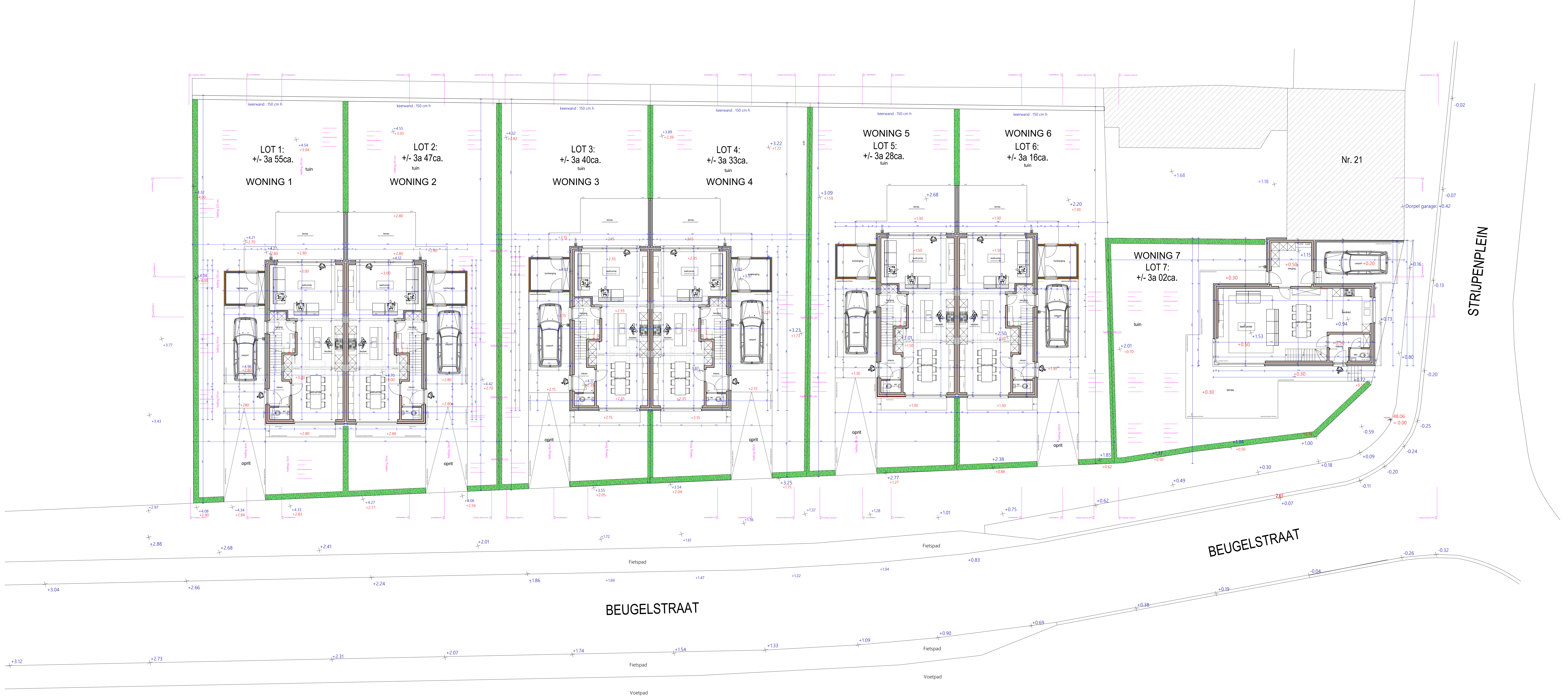
-- GRONDPLAN nieuw -- schaal 1/100 -- A0 -- afmetingen in cm
