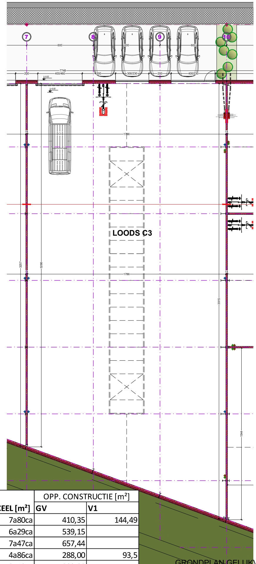
GRONDPLAN GELIJKVLOERS
