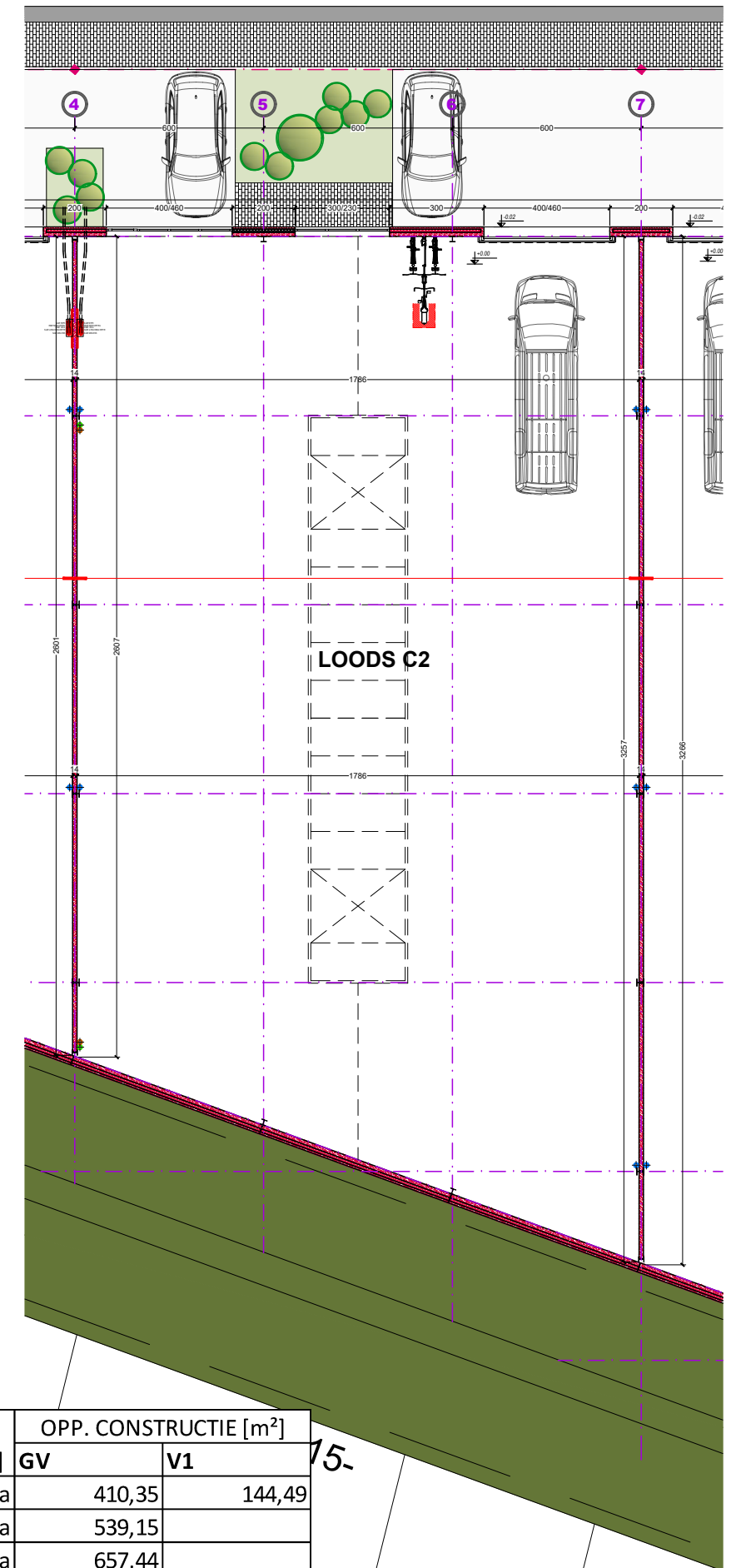
GRONDPLAN GELIJKVLOERS
