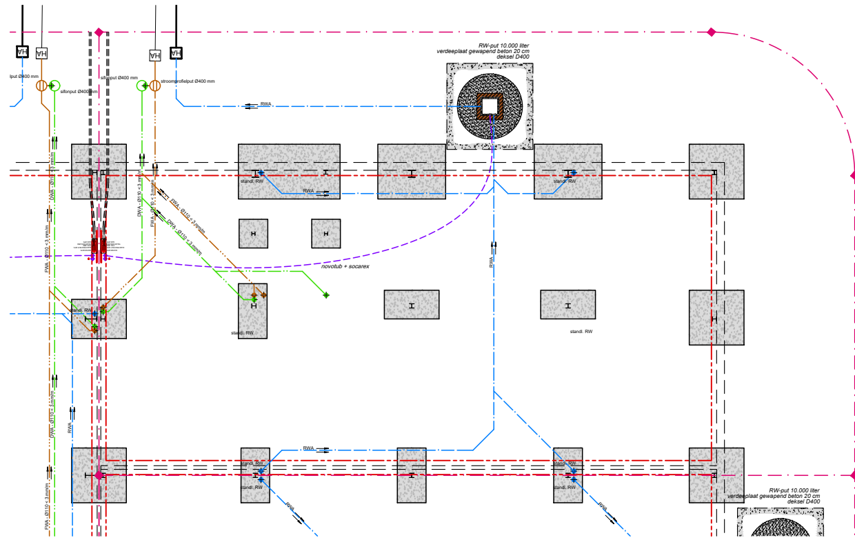
FUNDERINGEN & RIOLERINGEN
