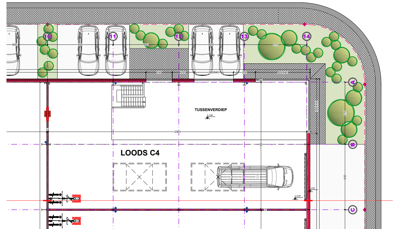
GRONDPLAN VERDIEPING
