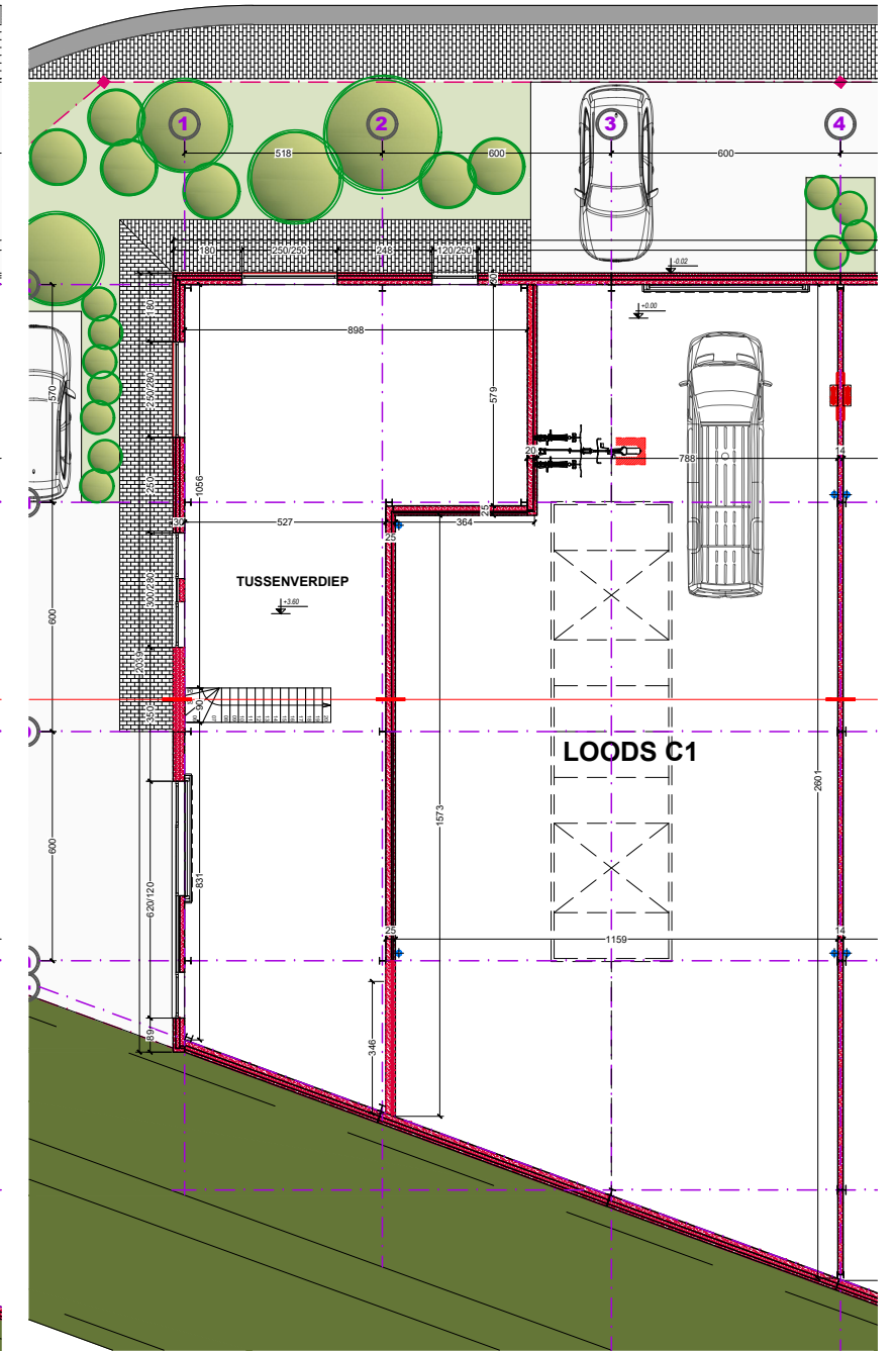
GRONDPLAN VERDIEPING
