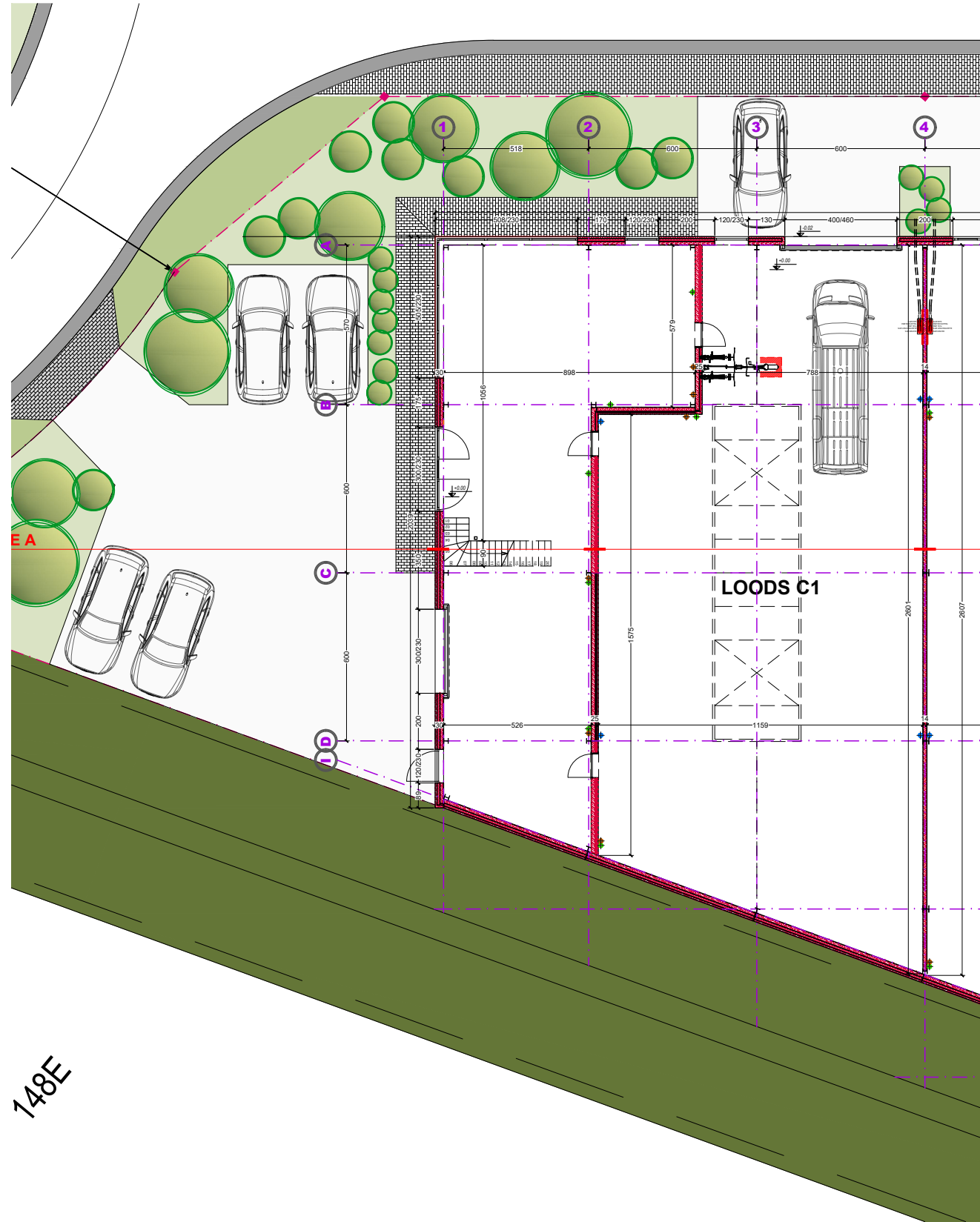
GRONDPLAN GELIJKVLOERS
