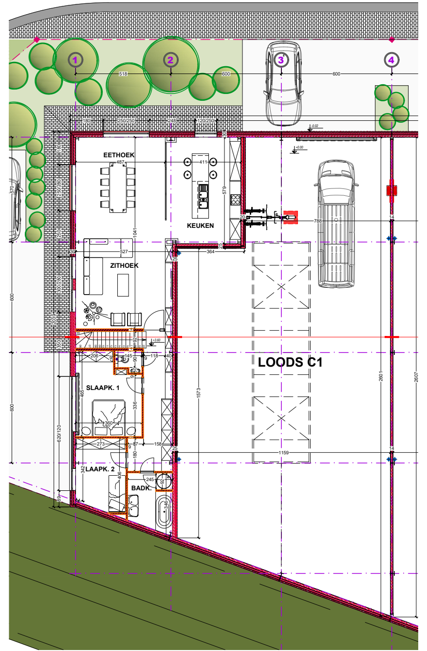
GRONDPLAN VERDIEPING
