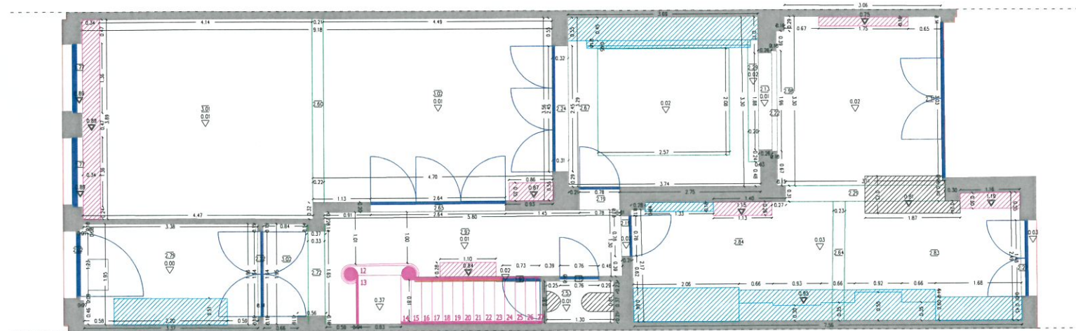
GELIJKVLOERSE VERDIEPING
