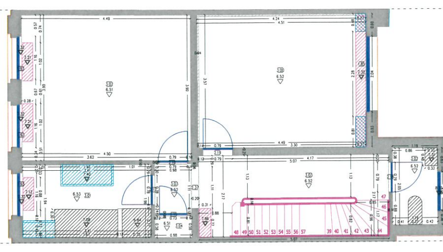
2DE VERDIEPING
