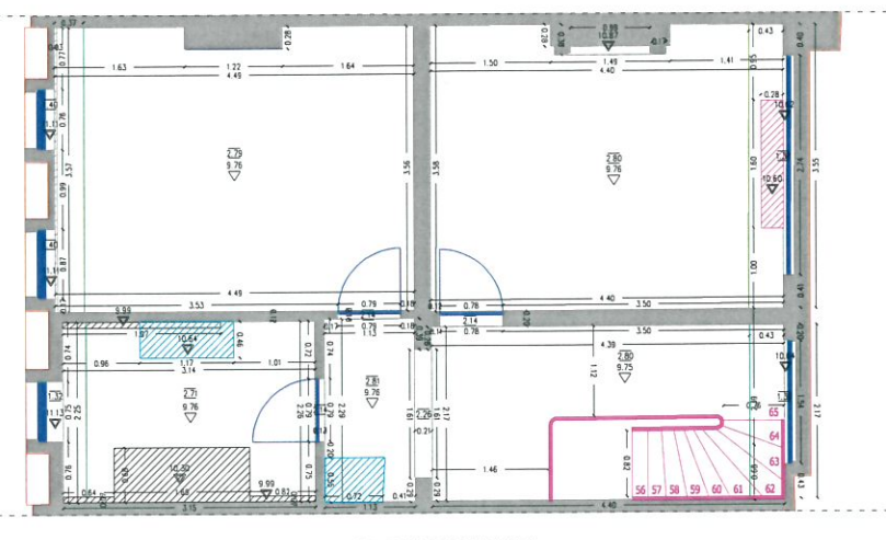
3DE VERDIEPING
