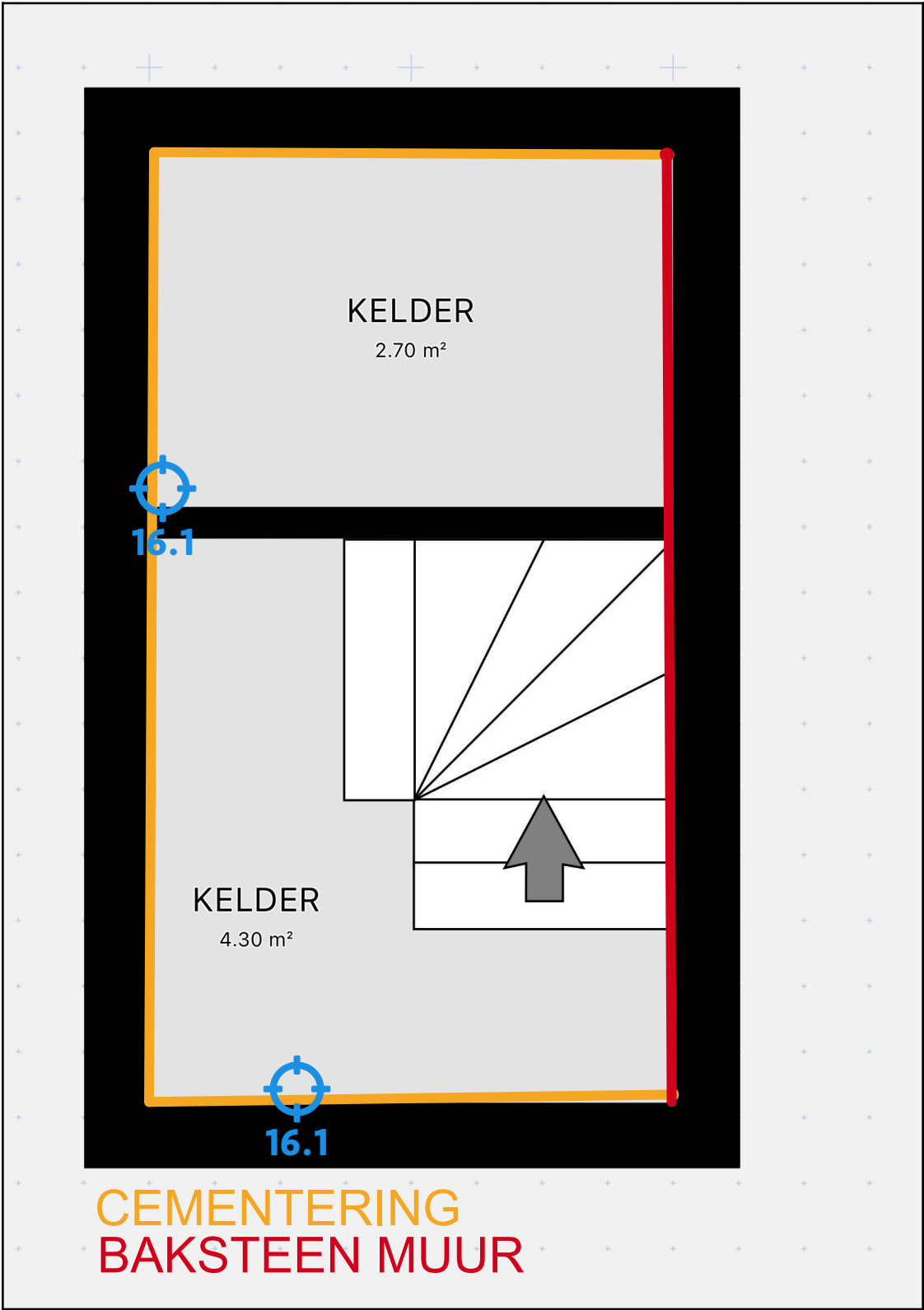
Legende van plan 1.1: Kelder
