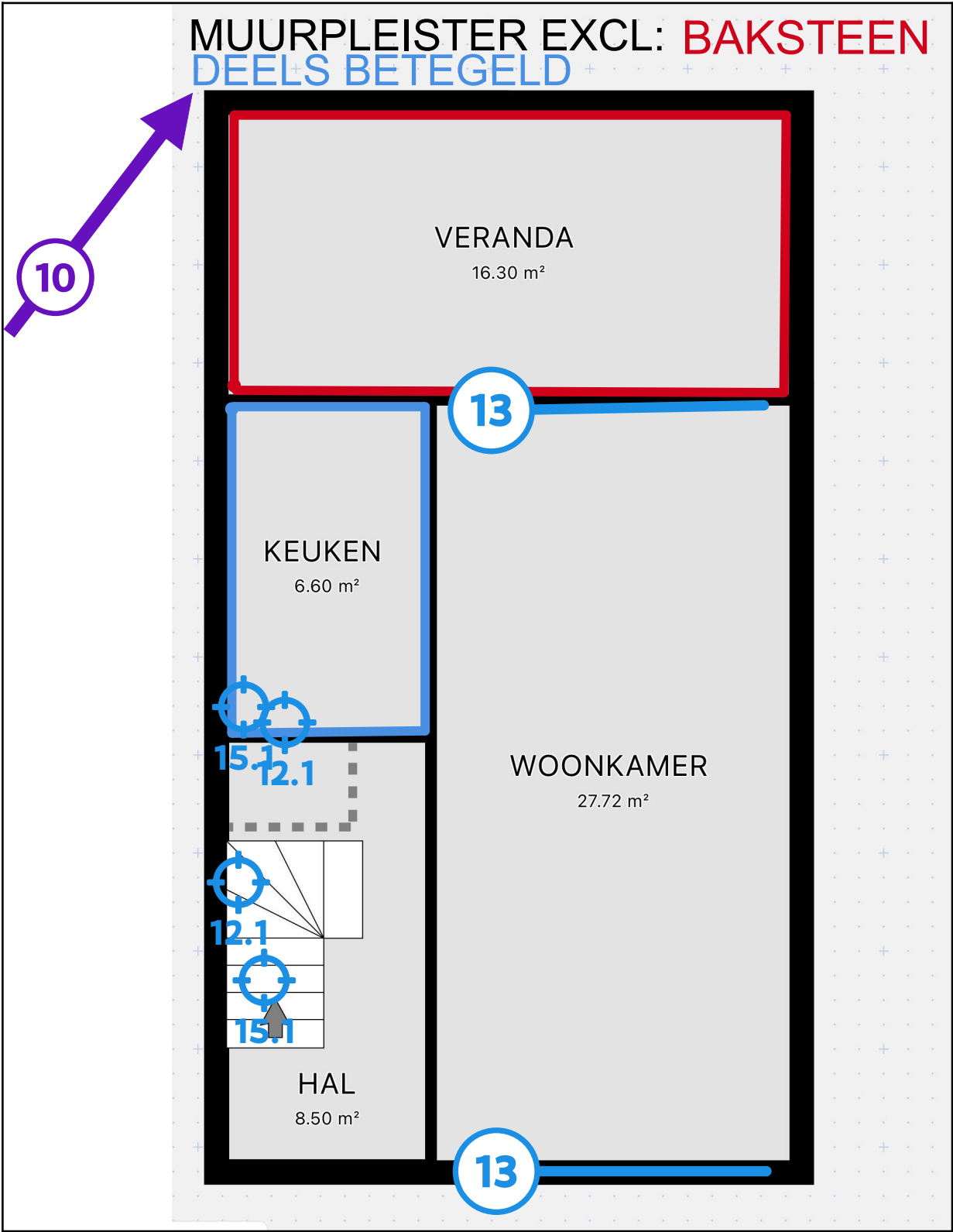
Legende van plan 1.3: Gelijkvloers
