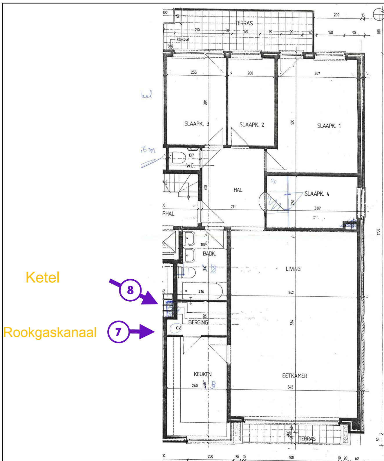
Legende van plan 1.5: Berging ketel/ rookgaskanaal
