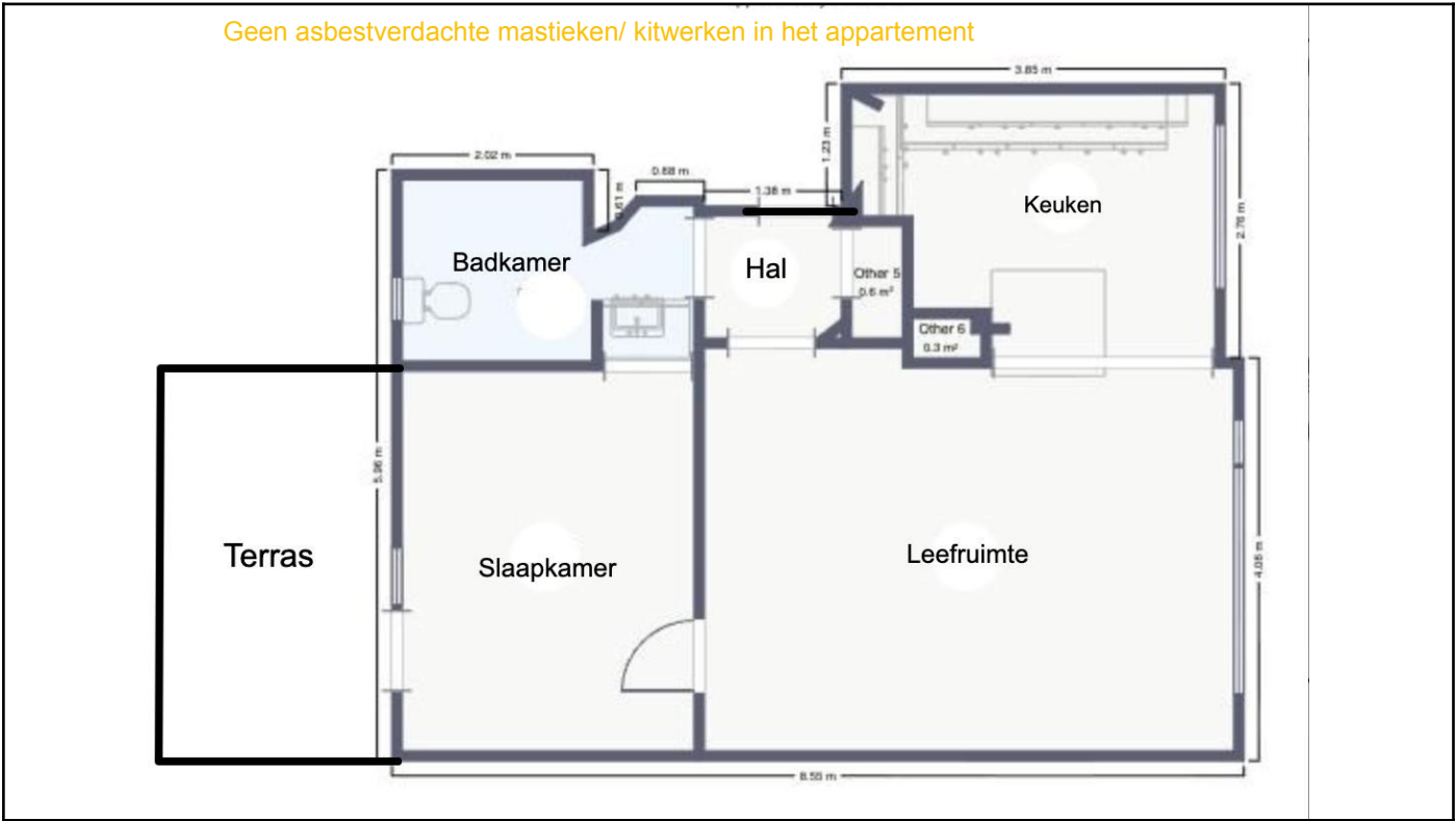
Legende van plan 1.8: Appartement mastieken / kitwerken
