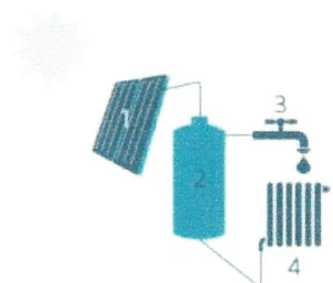
1 Zonnecollector | 2 Opslagvat zonneboiler 3 Sanitair warm water | 4 Afgegeven warmte voor ruimteverwarming (optioneel)
