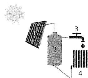
1 Zonnecollector 2 Opslagvat voor warm water 3 Douchewater 4 Radiator
