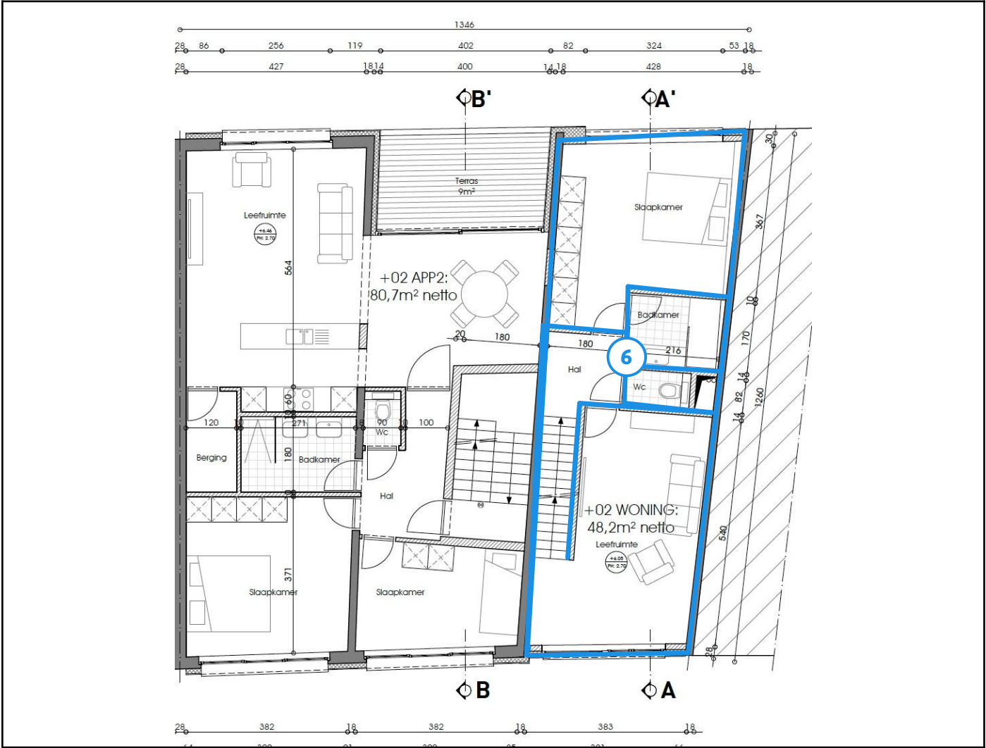
Legende van plan 1.4: 2de verdieping pleisterwerk wanden
