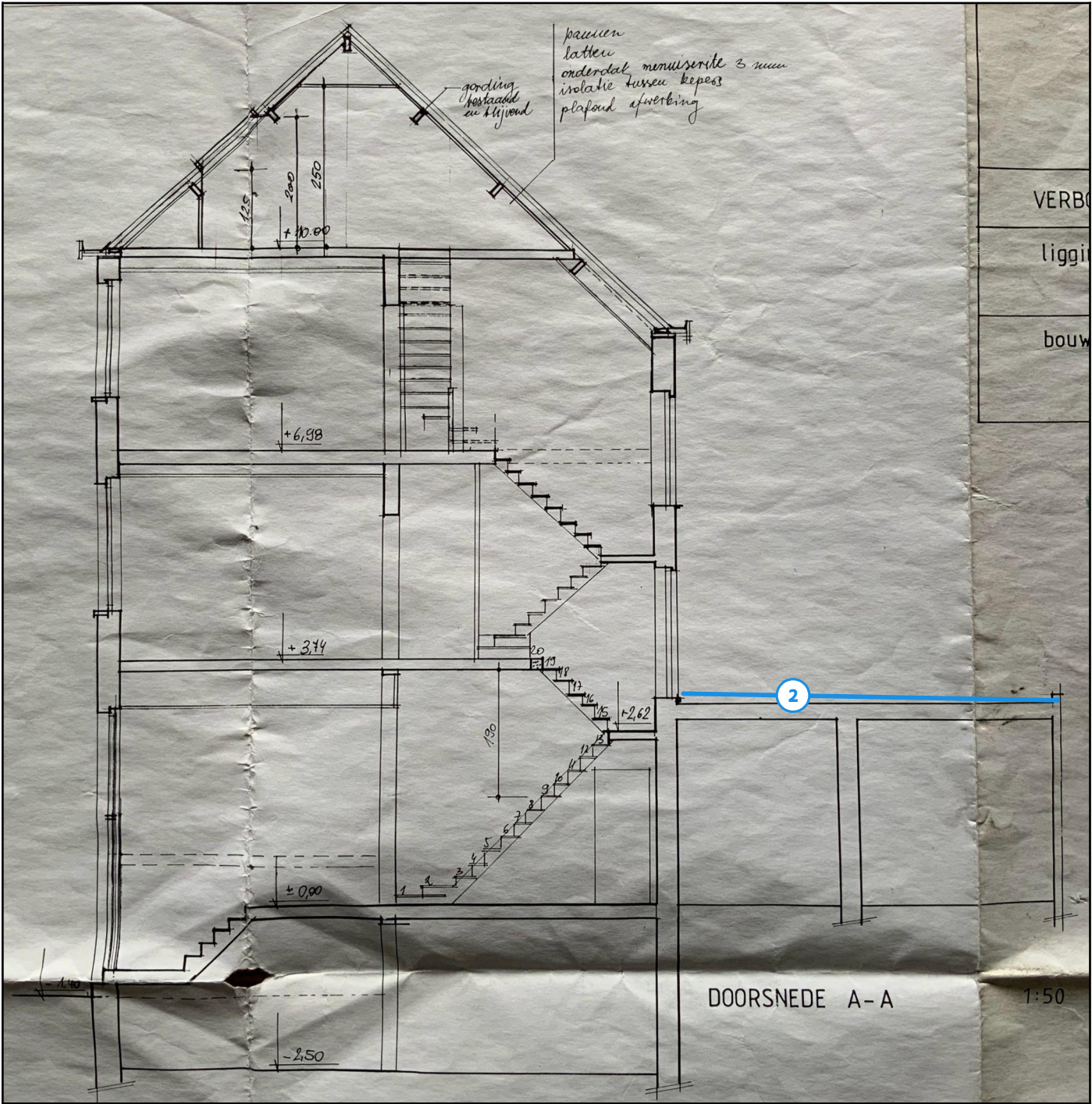
Legende van plan 1.3: doorsnede
