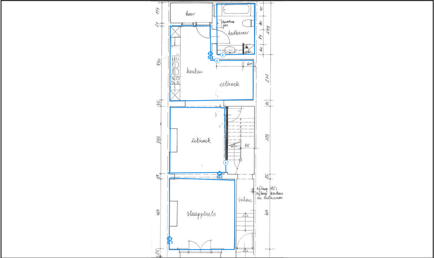
Legende van plan 1.1: plan gelijkvloersverdieping
