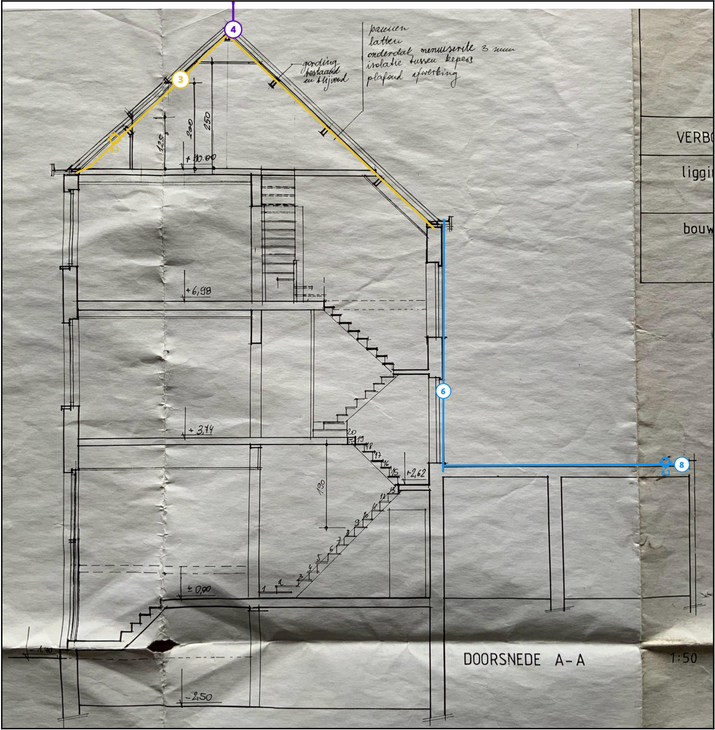
Legende van plan 1.1: doorsnede
