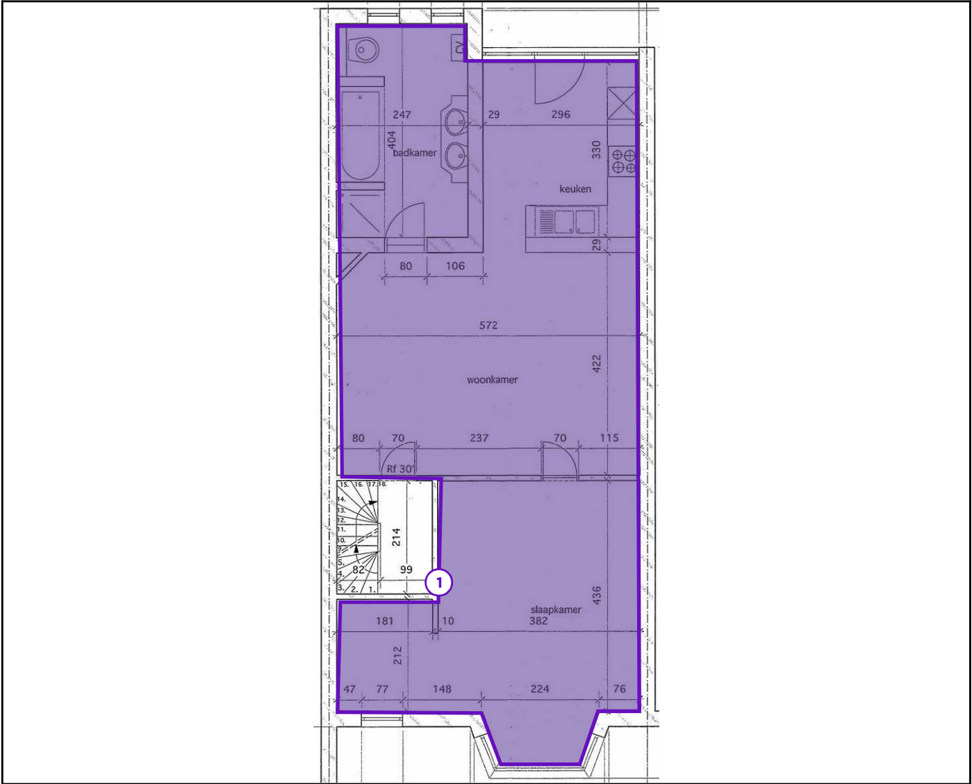
Legende van plan 1.3: Verdieping 1 plafond
