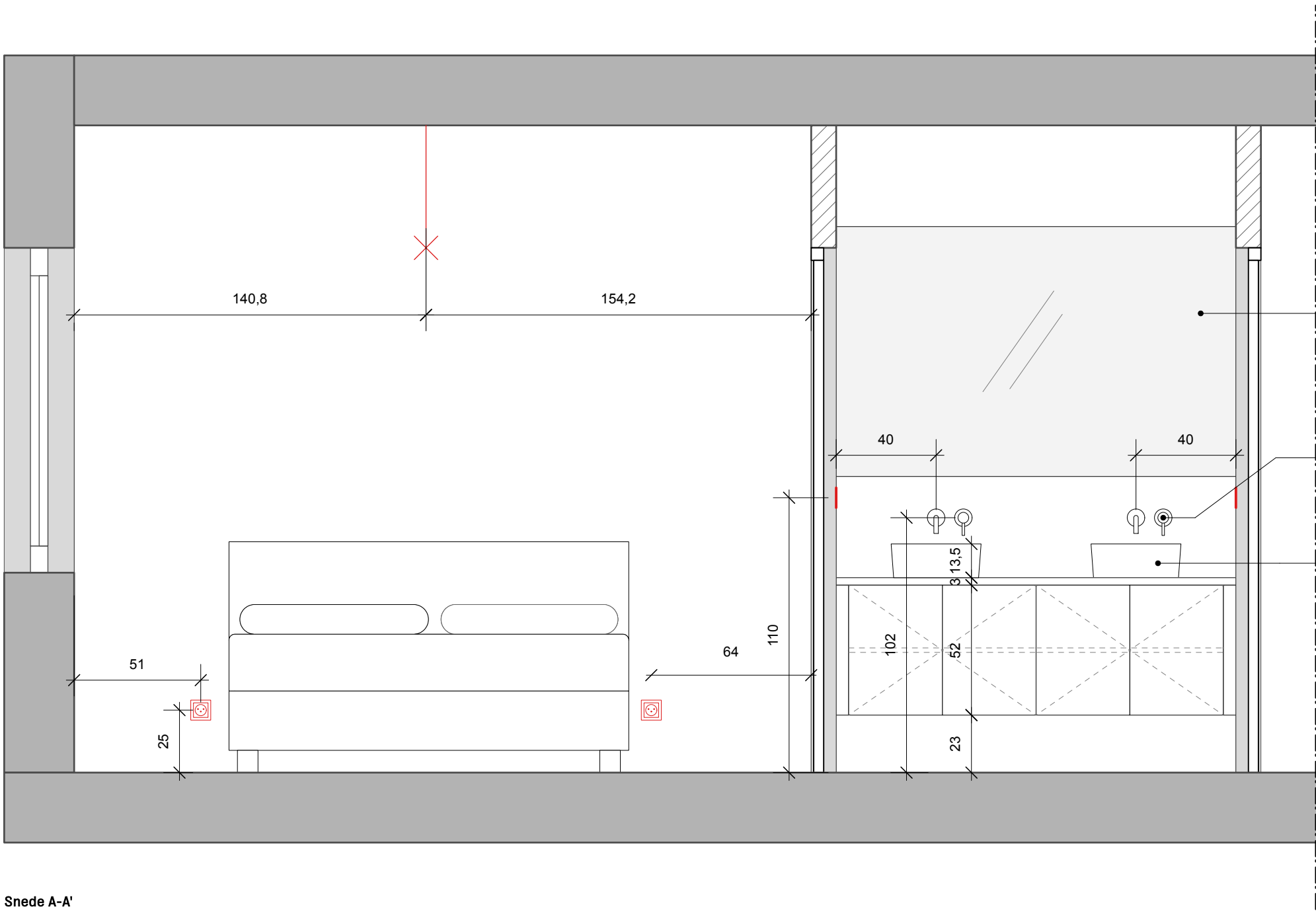
Snede A-A' slaapkamer 1 + badkamer
