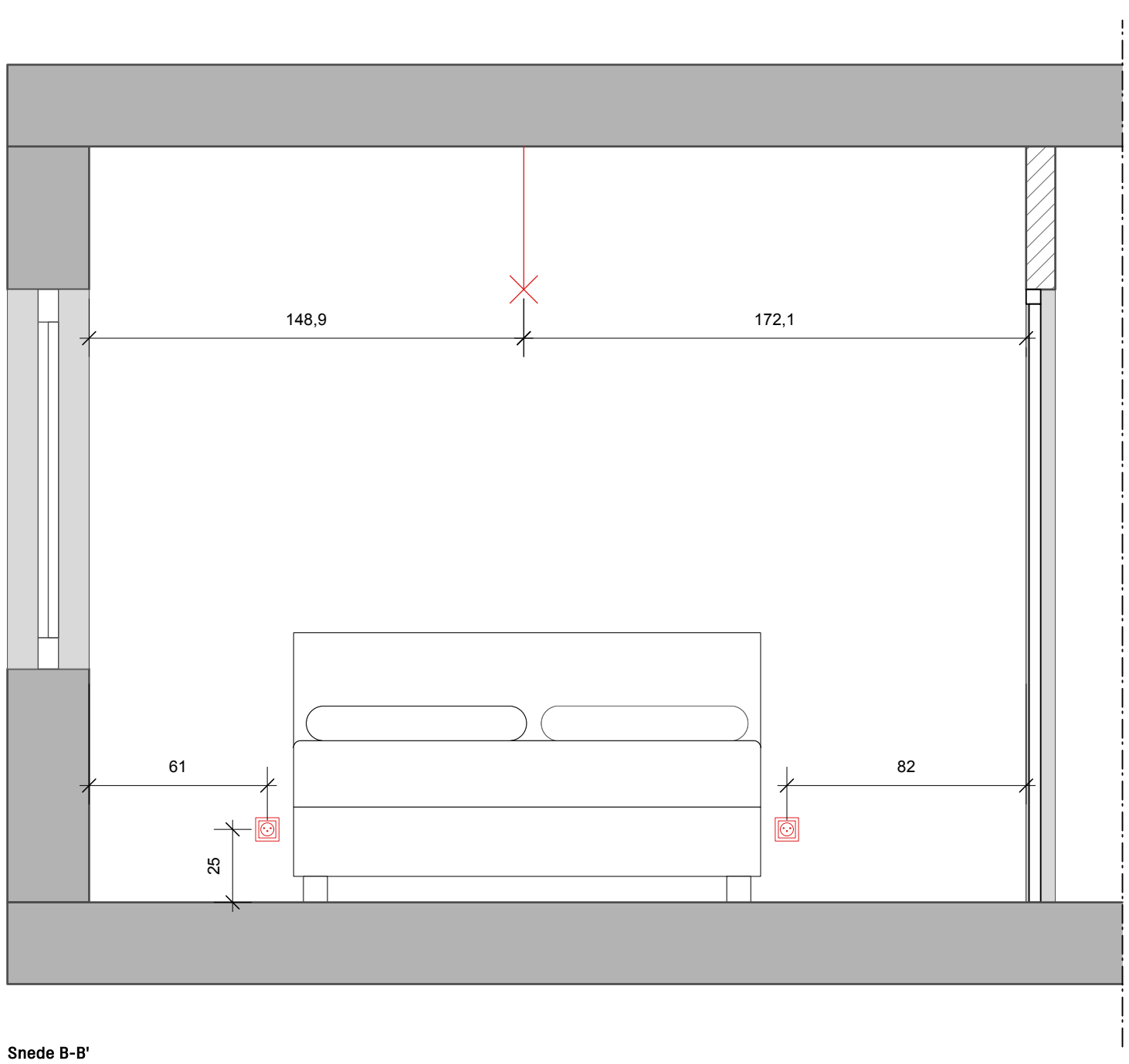
Snede B-B' slaapkamer 2
