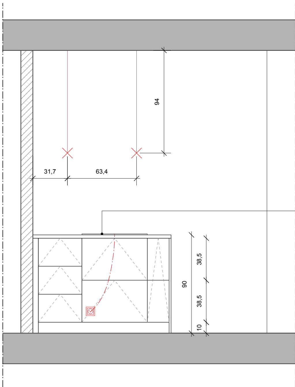
Snede D-D' keuken
