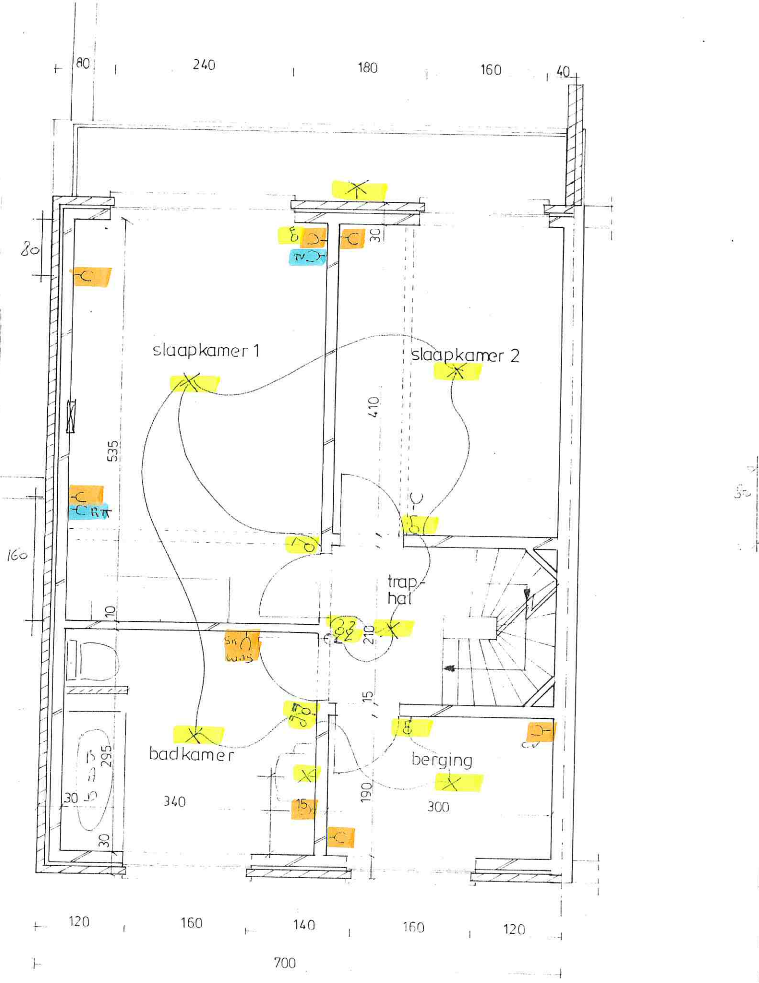
1 e Verdieping
