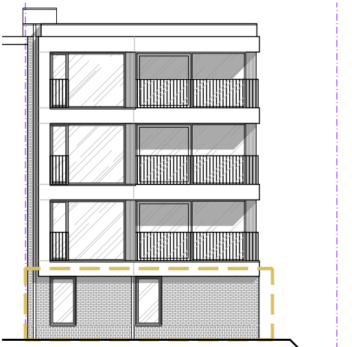
voorgevel
