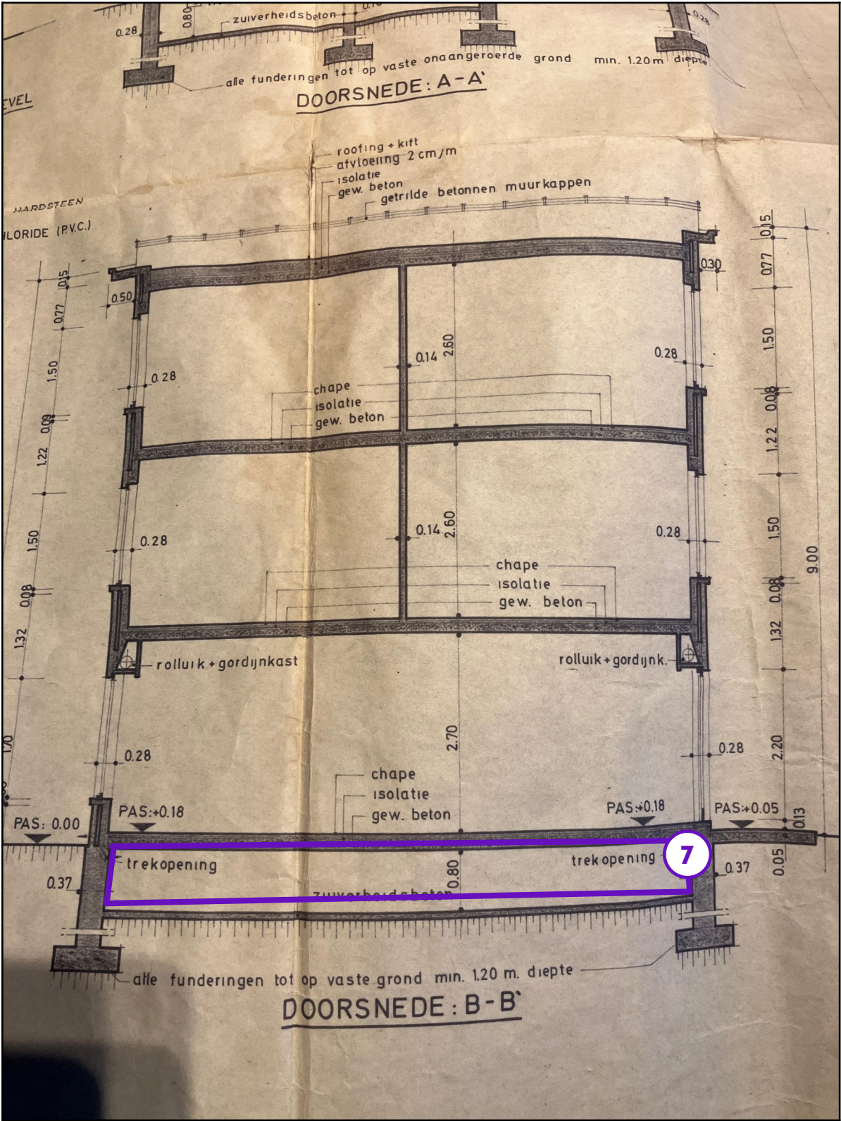
Legende van plan 1.6: Plan zijgevel - kruipruimte
