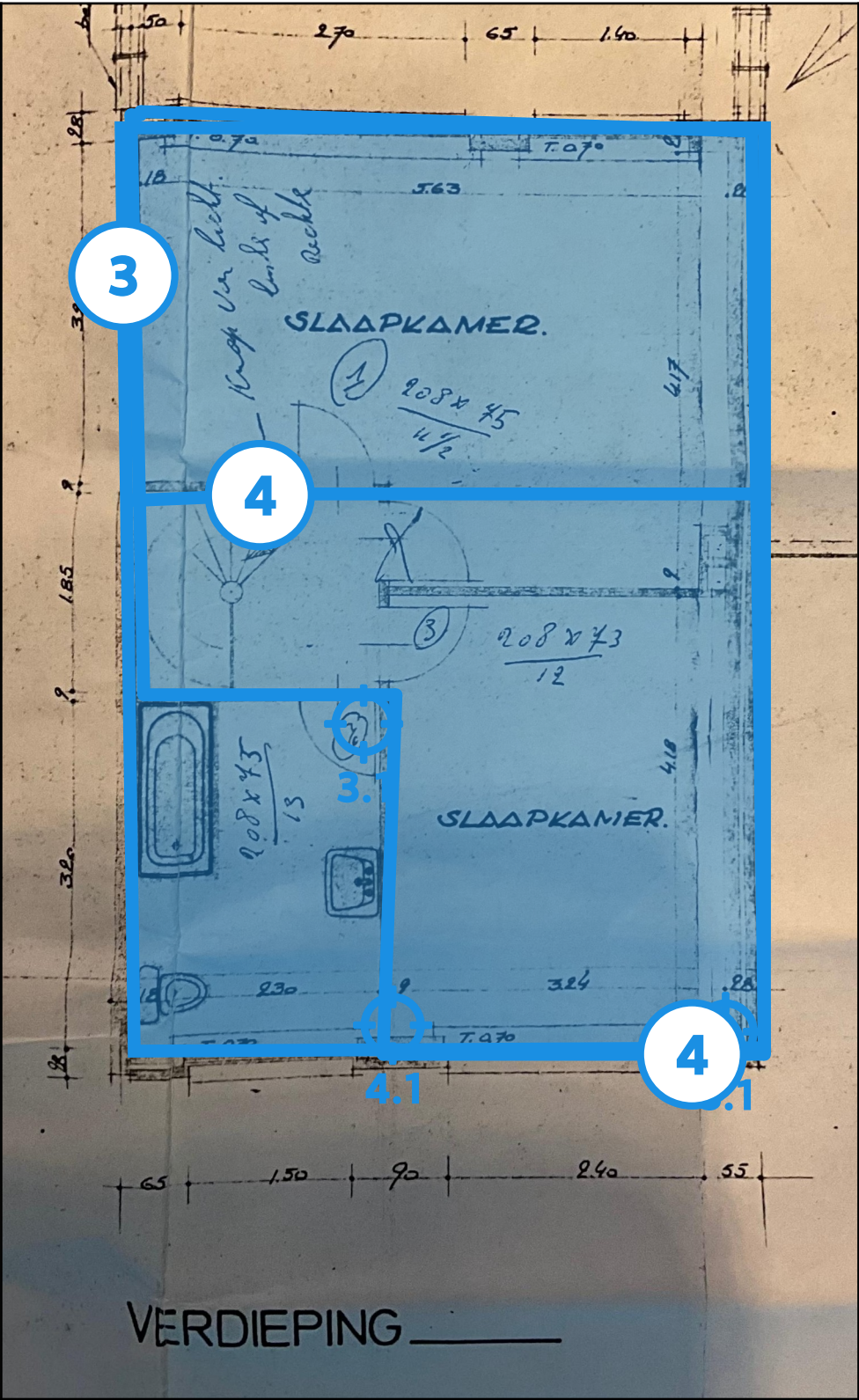
Legende van plan 1.2: 1e verdieping
