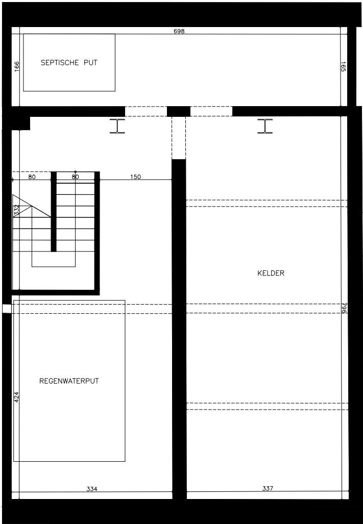
Grondplan
