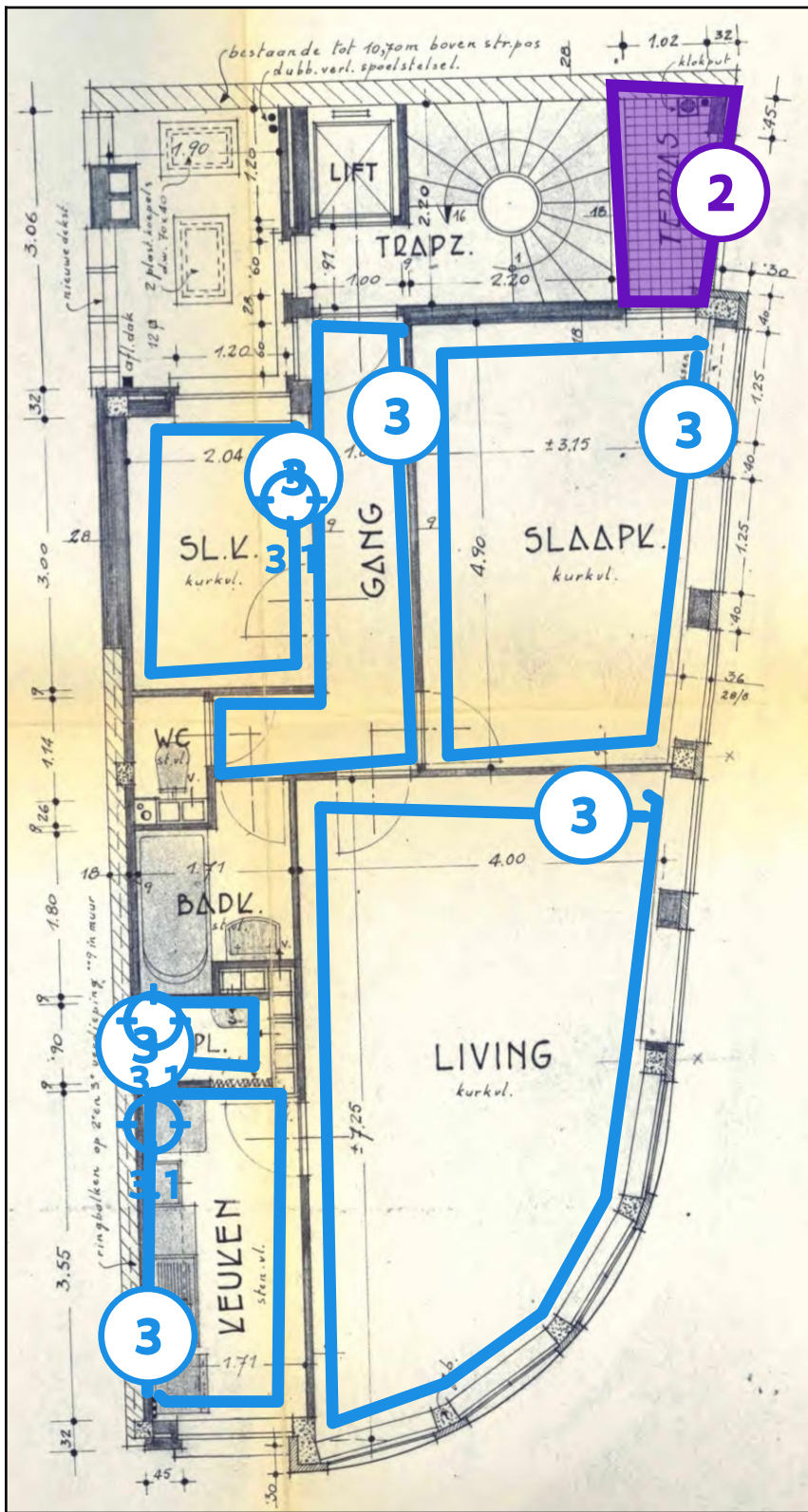
Legende van plan 1.1: Appartement 2
