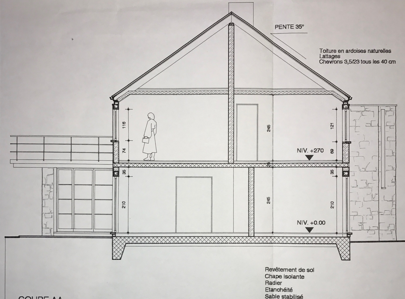
COUPE AA
