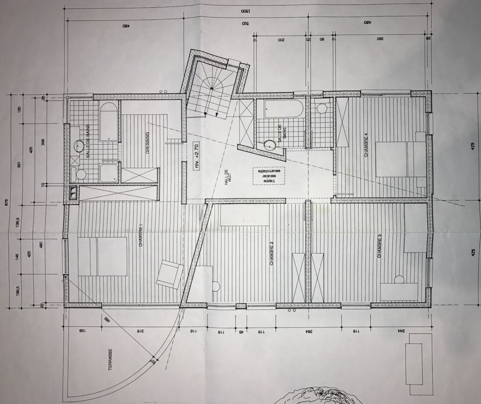
PLAN ETAGE
